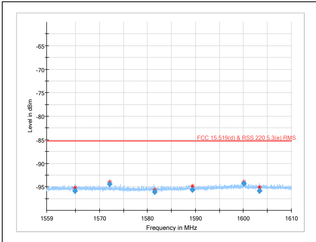
Plot 38: 1559 MHz to 1610 MHz §15.519 (d), UWB test mode
