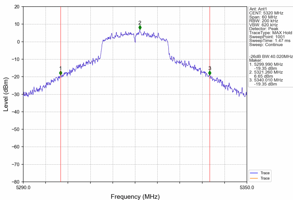
802.11ac(VHT20) HCH 5320MHz Ant1 NTV
