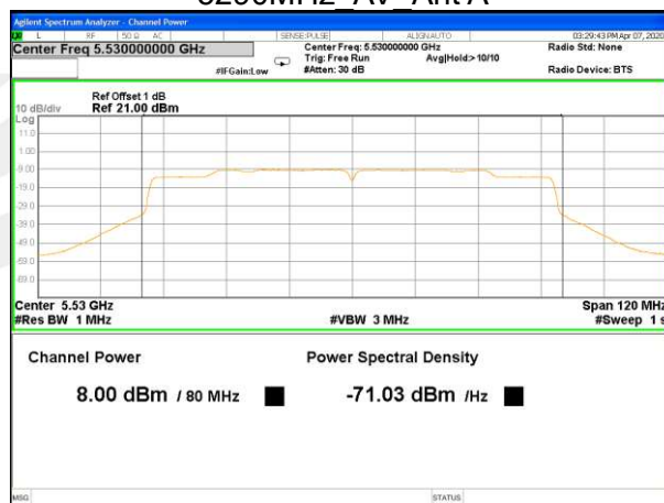
5530MHz_AV_Ant A
