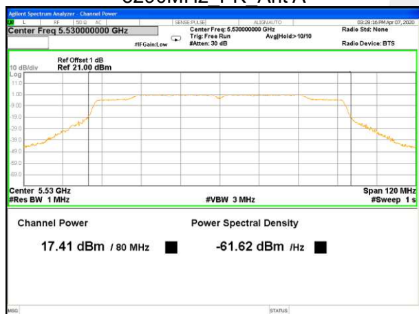
5530MHz_PK_Ant A
