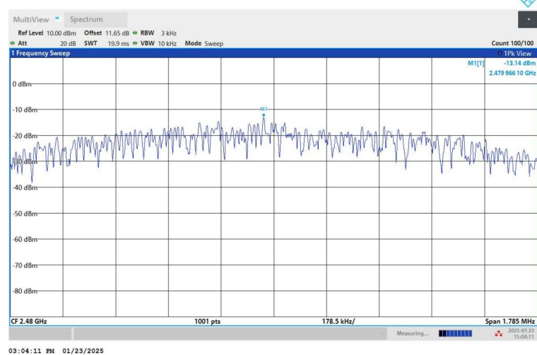
BLE_2M_Ant1_2480
