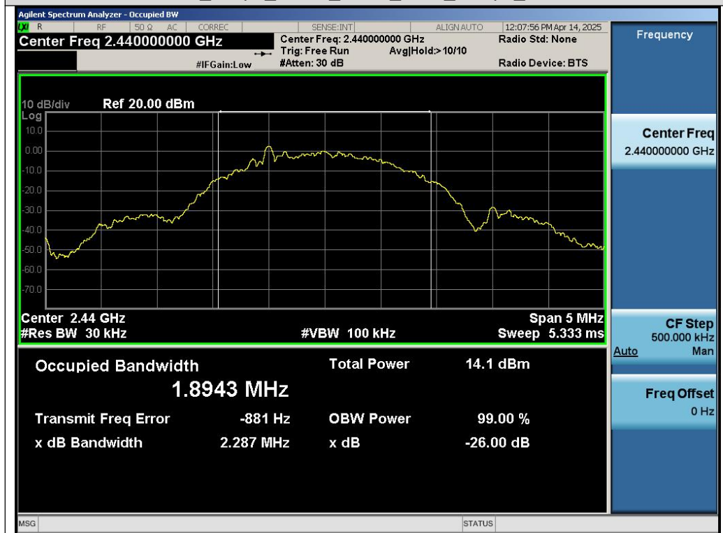
Test_Graph_GFSK_ANT1_2440_2Mbps_OBW
