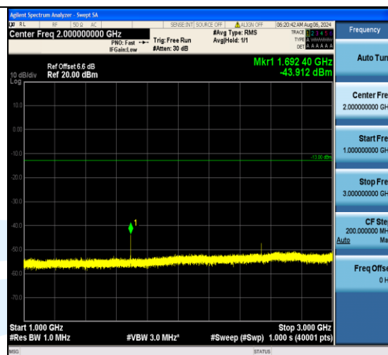
Band5 3MHz QPSK 20635 1RB#0 1000~3000 1000~3000
