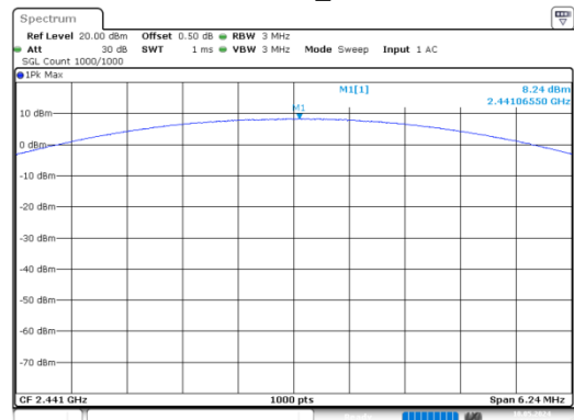
\pi/4 -DQPSK_Middle
