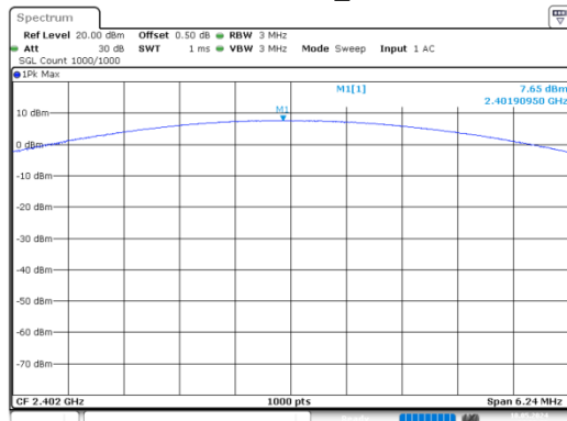
\pi/4 -DQPSK_Low
