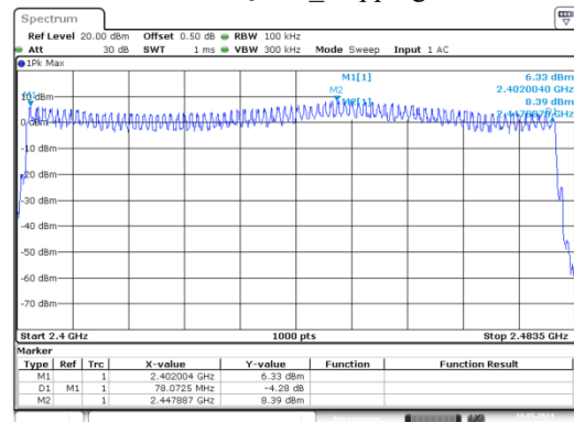
\pi/4 -DQPSK_Hopping
