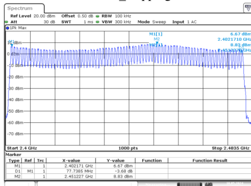
GFSK_Hopping
