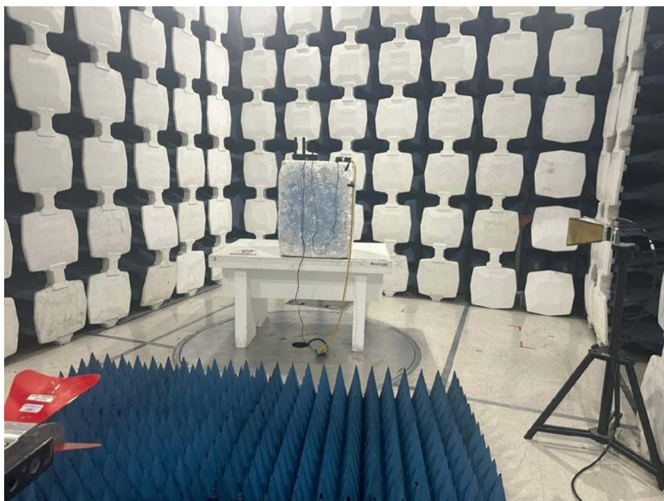
1-18GHz Front
