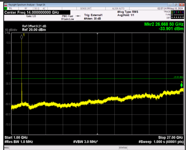
41-41-5MHz-20MHz-QPSK-QPSK-40528-40645-1RB#0-1RB#99-1000~27000MHz-PASS
