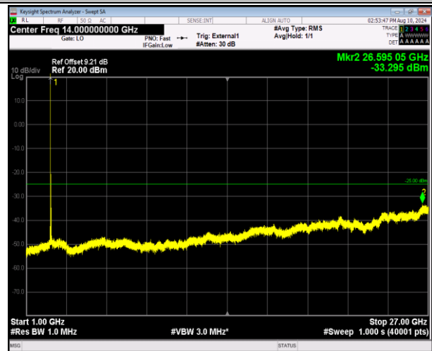
41-41-5MHz-20MHz-QPSK-QPSK-40528-40645-1RB#0-ORB#0-1000~27000MHz-PASS
