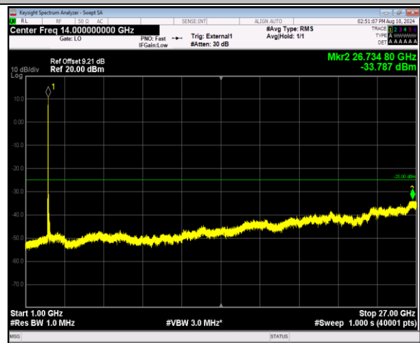
41-41-5MHz-20MHz-16QAM-16QAM-39683-39800-1RB#0- 1RB#99-1000~27000MHz-PASS
