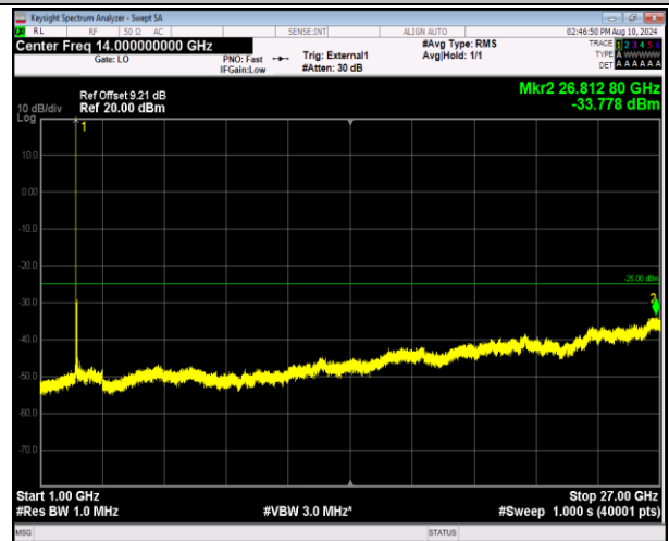
41-41-5MHz-20MHz-QPSK-QPSK-39683-39800-1RB#0-0R B#0-1000~27000MHz-PASS
