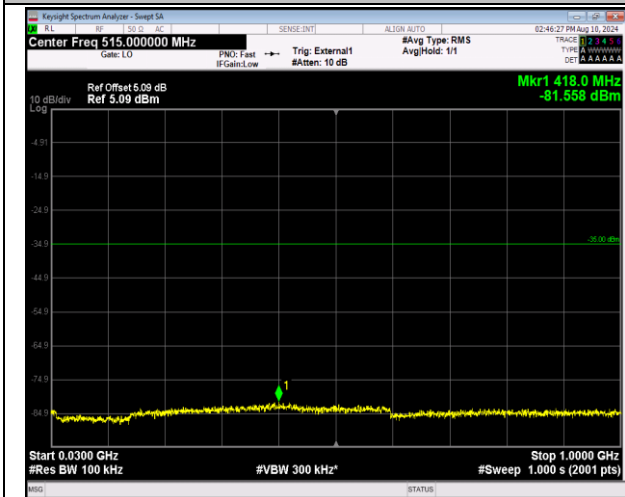
41-41-5MHz-20MHz-QPSK-QPSK-39683-39800-1RB#0-0- ORB#0-30~1000MHz-PASS
