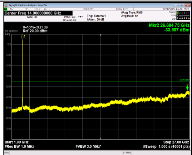
41-41-5MHz-20MHz-QPSK-QPSK-40528-40645-25RB#0-100RB#0-1000~27000MHz-PASS
