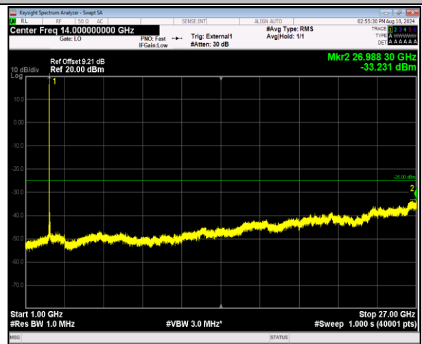
41-41-5MHz-20MHz-QPSK-QPSK-40528-40645-1RB#24-0RB#0-1000~27000MHz-PASS
