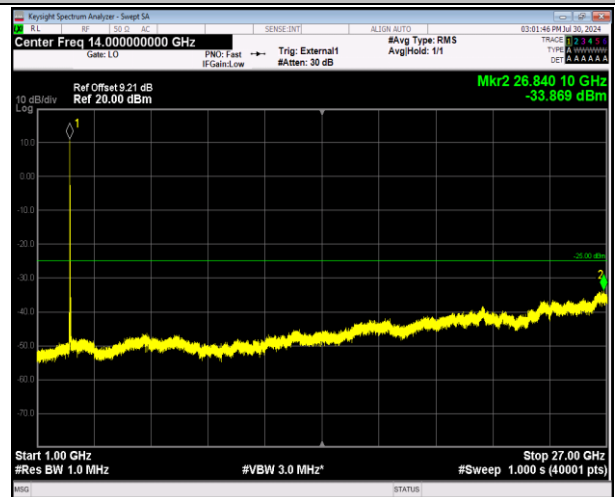
41-41-5MHz-20MHz-64QAM-64QAM-39683-39800-1RB#0- 1RB#99-1000~27000MHz-PASS
