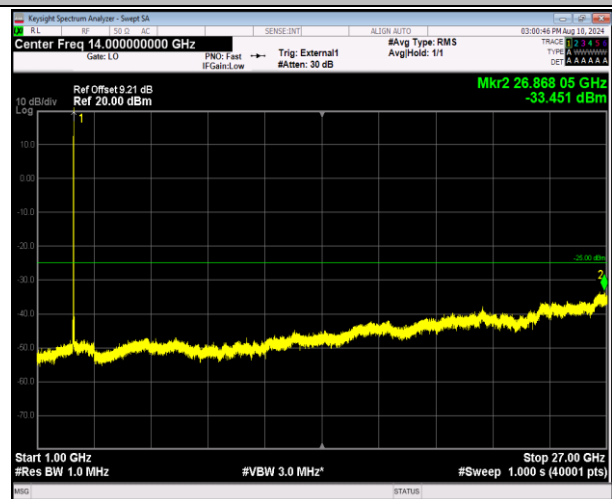
41-41-5MHz-20MHz-QPSK-QPSK-41373-41490-1RB#0-0R B#0-1000~27000MHz-PASS
