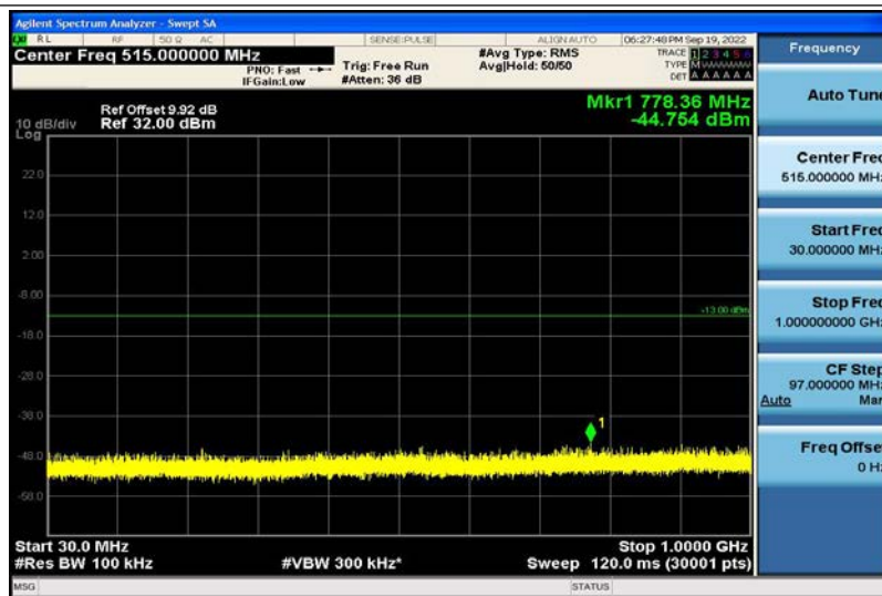
Band4-3MHz-QPSK-19965-1RB#0-30~1000MHz
