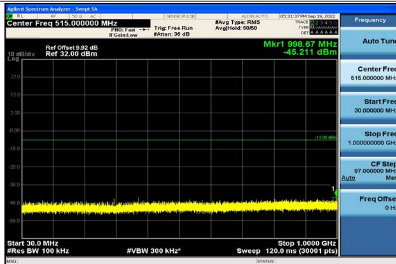
Band2-20MHz-16QAM-18900-1RB#0-30~1000MHz
