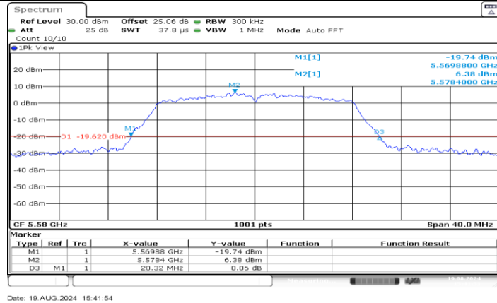
11A_Ant1_5580
