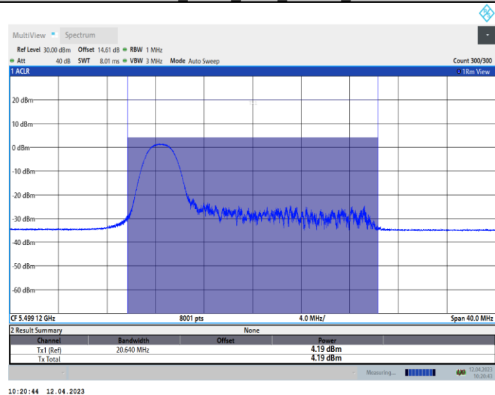
11AX20_Ant10_5500_52Tone_RU37
