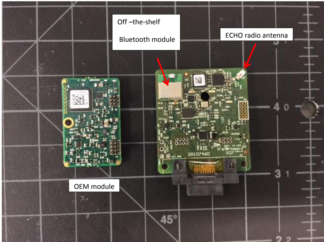
PCBAs
