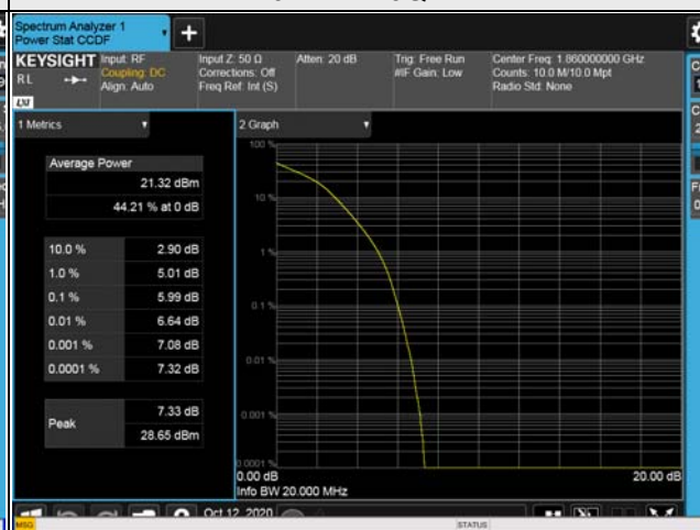
20MHz / 16QAM
