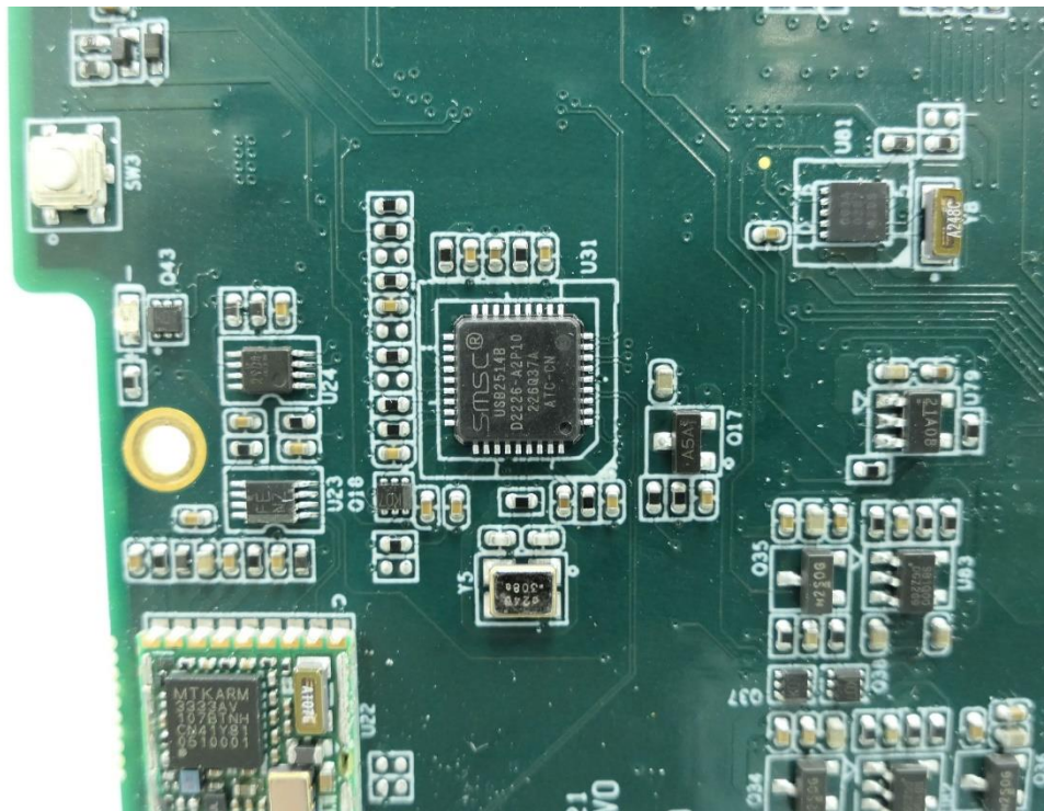
(20) EUT Photo
