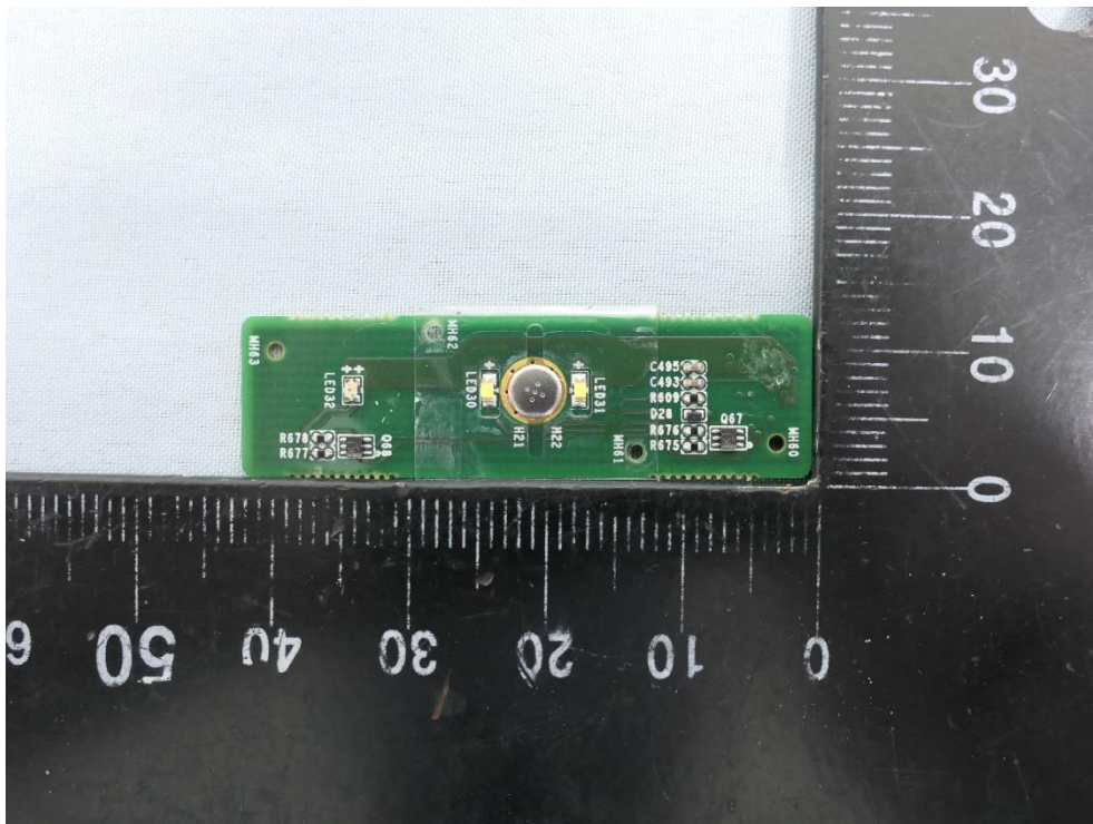
(44) EUT Photo
