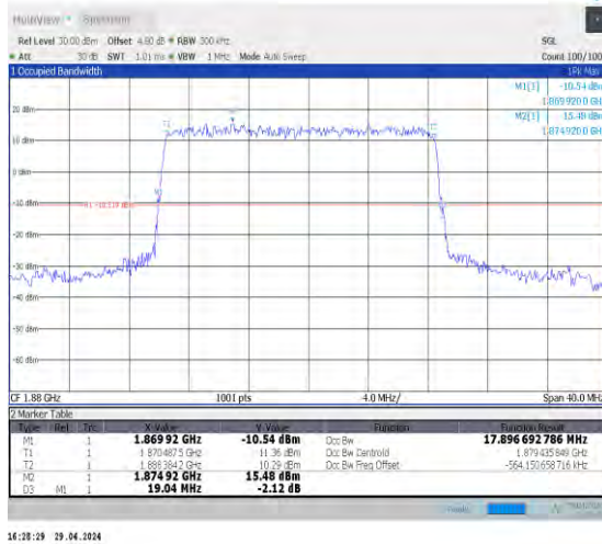
1-N2-15-20-M-2-DFT-PI2BPSK-Outet_Full-100@0-A nt0-17.897-19.040-≤20-PASS
