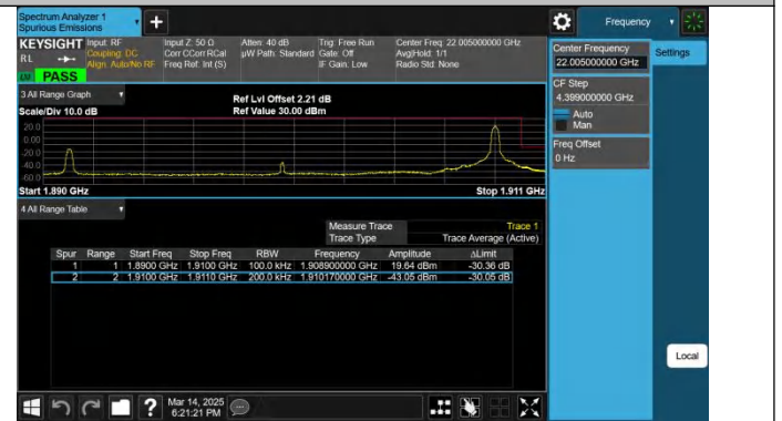
Band2-20MHz-QPSK-19100-1RB#99-PASS
