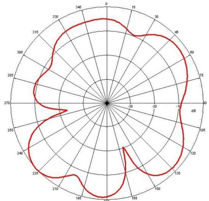
E-PLANE
