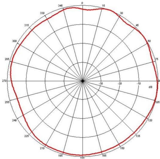
H-PLANE
