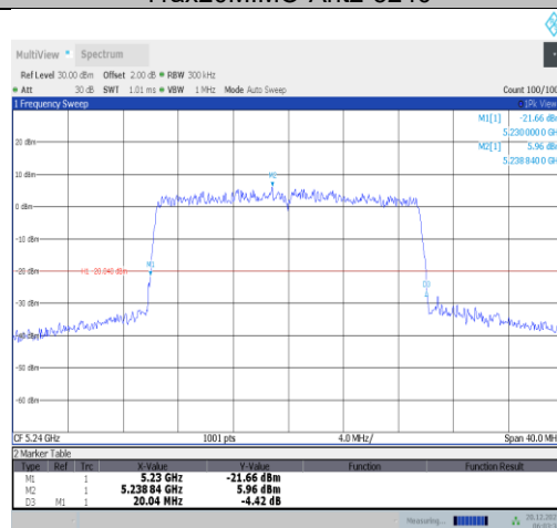
11ax20MIMO-Ant4-5240
