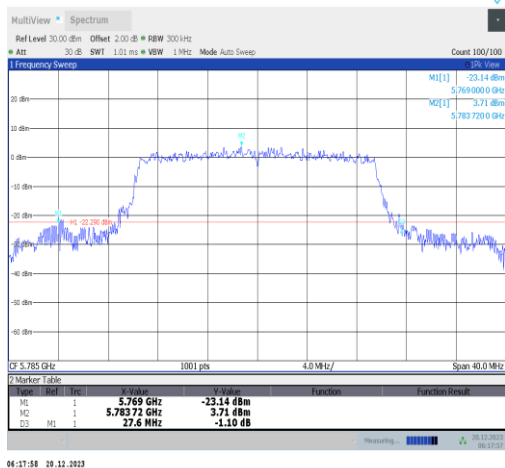
11ax20MIMO-Ant3-5785
