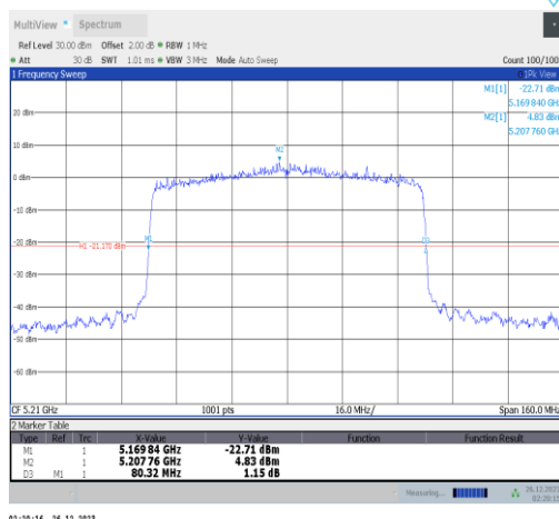
11ax80MIMO-Ant1-5210
