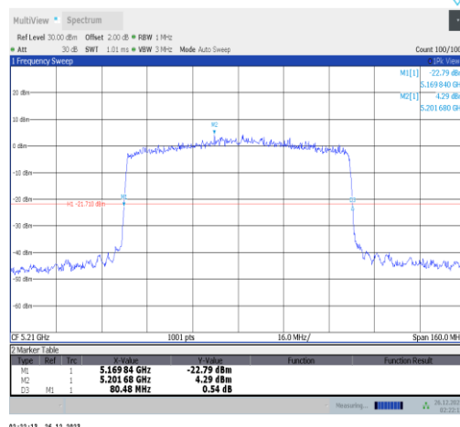
11ax80MIMO-Ant2-5210
