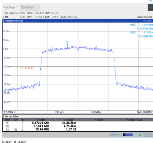
11ax40MIMO-Ant1-5190
