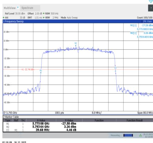
11ax40MIMO-Ant1-5795
