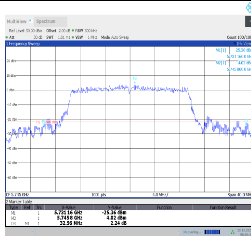
11ax20MIMO-Ant4-5745
