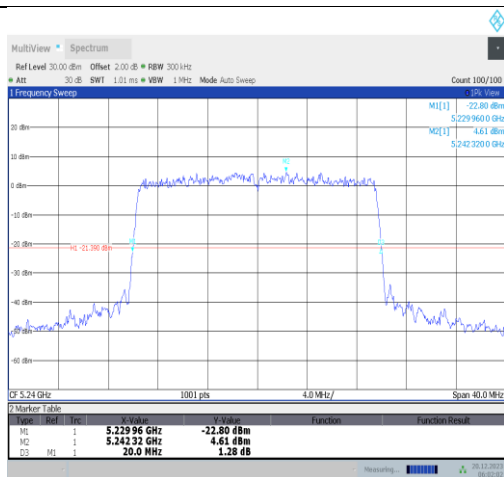
11ax20MIMO-Ant1-5240
