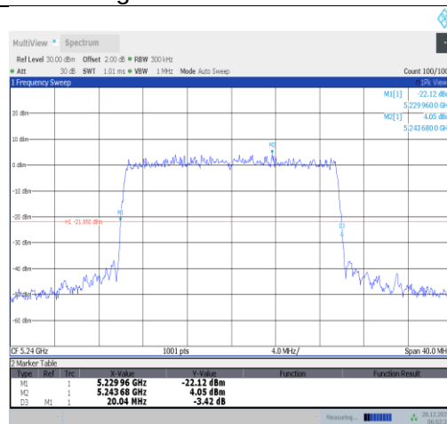
11ax20MIMO-Ant2-5240
