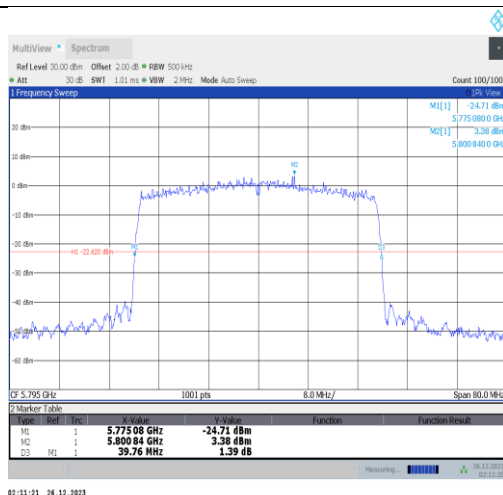
11ax40MIMO-Ant3-5795
