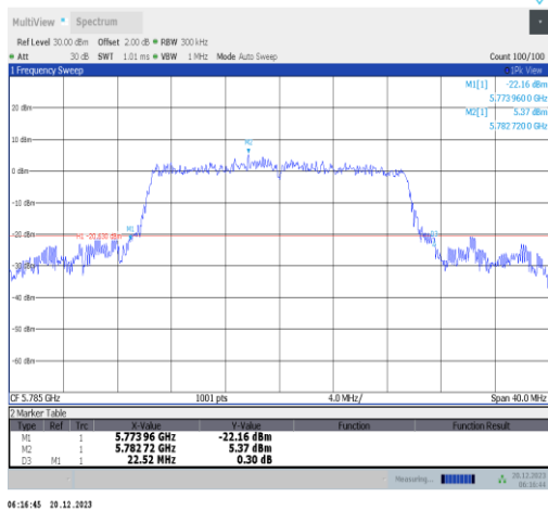
11ax20MIMO-Ant1-5785
