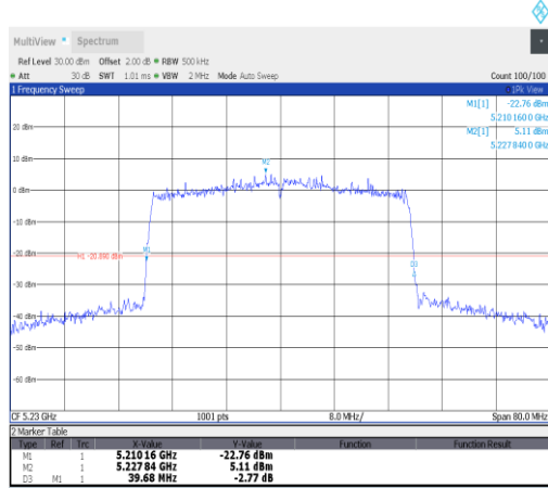
11ax40MIMO-Ant3-5230
