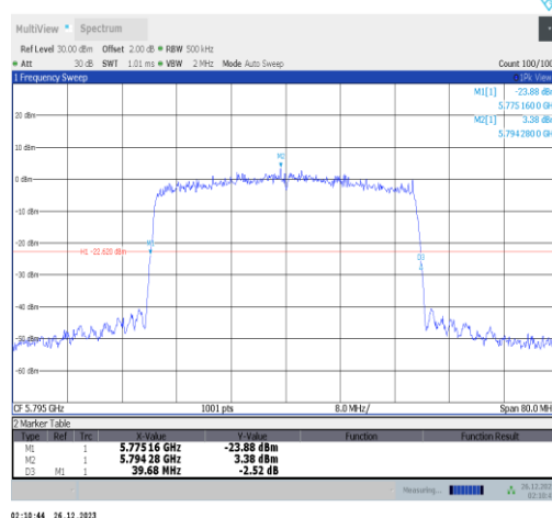
11ax40MIMO-Ant2-5795
