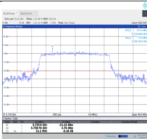
11ax20MIMO-Ant1-5745
