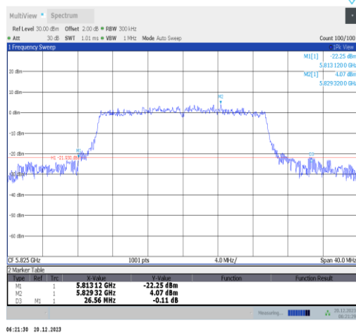
11ax20MIMO-Ant4-5825
