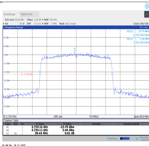
11ax40MIMO-Ant1-5755
