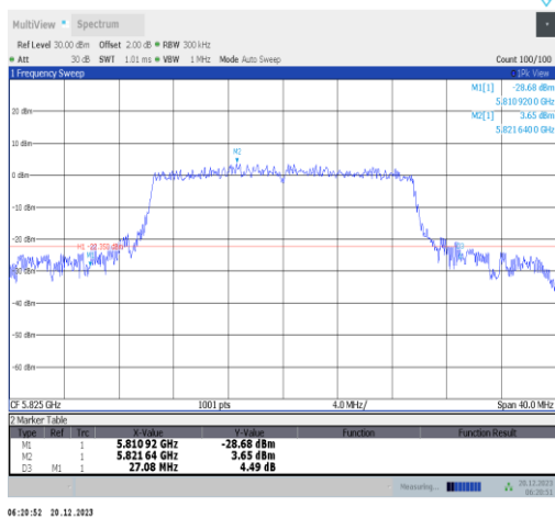
11ax20MIMO-Ant3-5825
