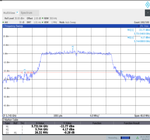
11ax20MIMO-Ant3-5745
