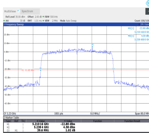
11ax40MIMO-Ant4-5230
