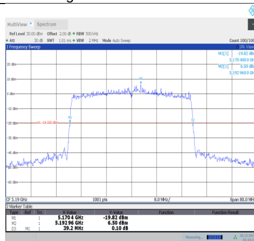
11ax40MIMO-Ant4-5190
