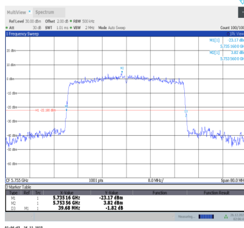
11ax40MIMO-Ant4-5755
