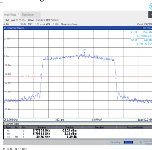
11ax40MIMO-Ant4-5795
