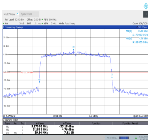
11ax40MIMO-Ant3-5190
