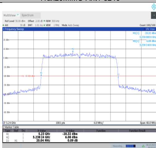
11ax20MIMO-Ant3-5240
