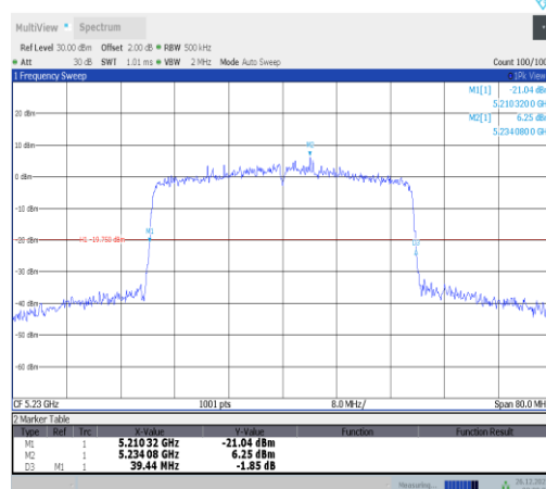
11ax40MIMO-Ant2-5230
