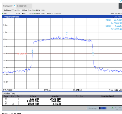
11ax80MIMO-Ant3-5210
