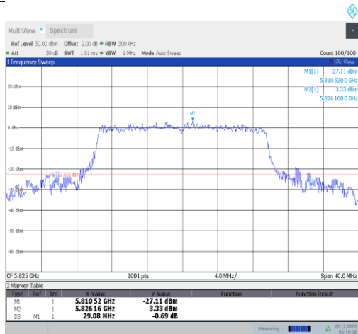
11ax20MIMO-Ant1-5825
