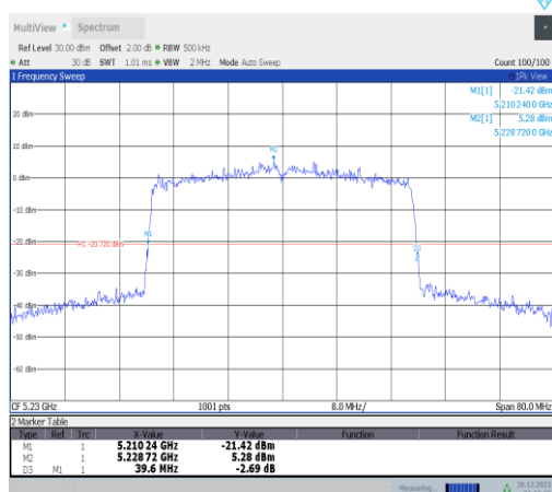
11ax40MIMO-Ant1-5230
