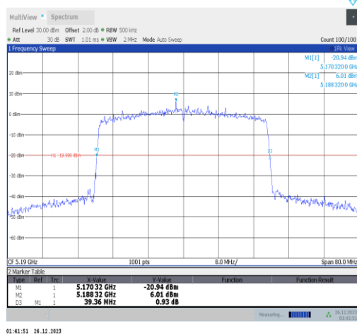
11ax40MIMO-Ant2-5190
