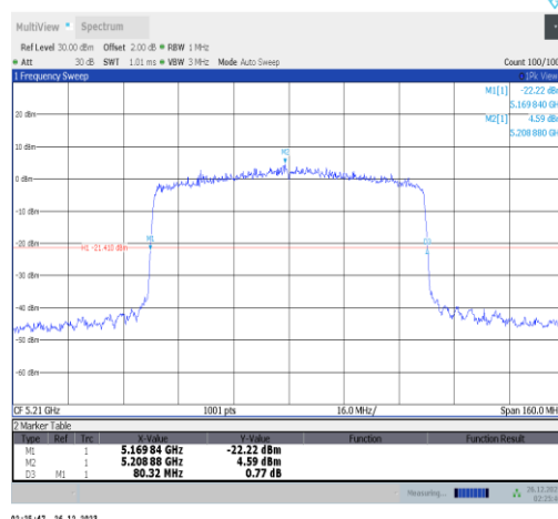
11ax80MIMO-Ant4-5210
