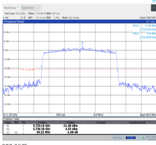
11ax40MIMO-Ant3-5755
