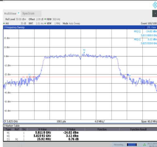
11ax20MIMO-Ant2-5825
