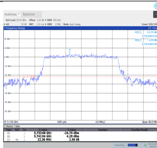
11ax20MIMO-Ant2-5745
