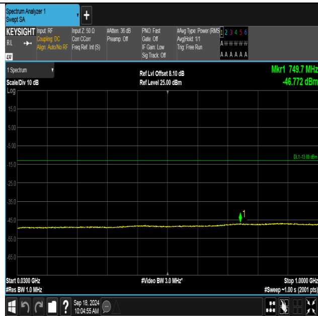
Band2-9400-3-30~1000MHz-PASS
