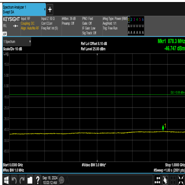
Band2-9538-2-30~1000MHz-PASS
