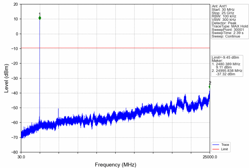
GFSK_DH5_HOPP_Ant1_NTNV
