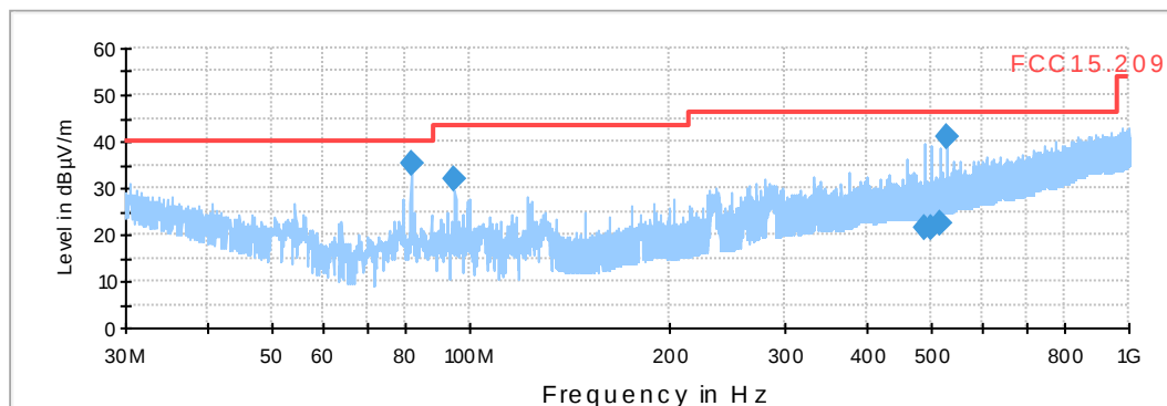
01_FCC15.209_hor+vert_KP0
