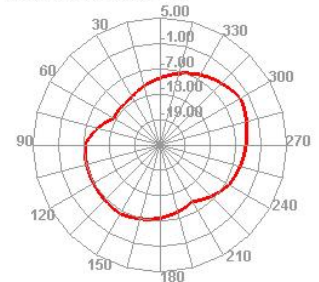
5150.000MHz H
