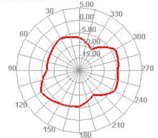
5150.000MHz E2
