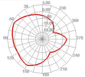
5800.000MHz E1
