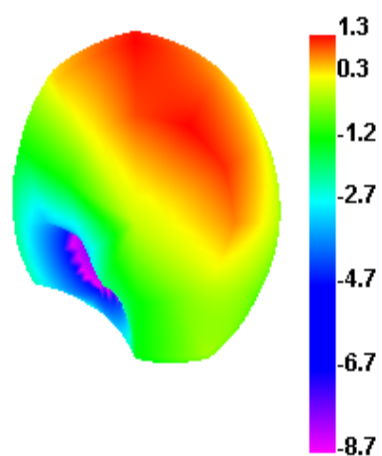
2500.000MHz E1
