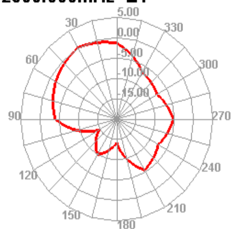
2500.000MHz E1
