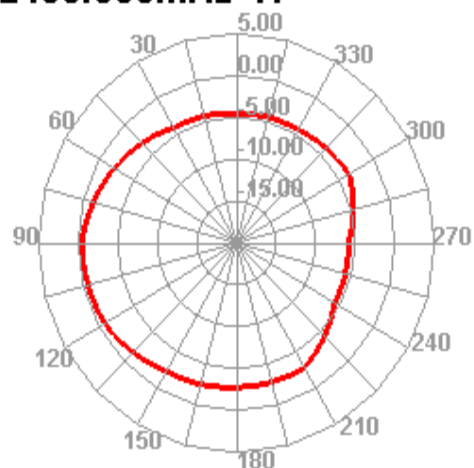
2450.000MHz H
