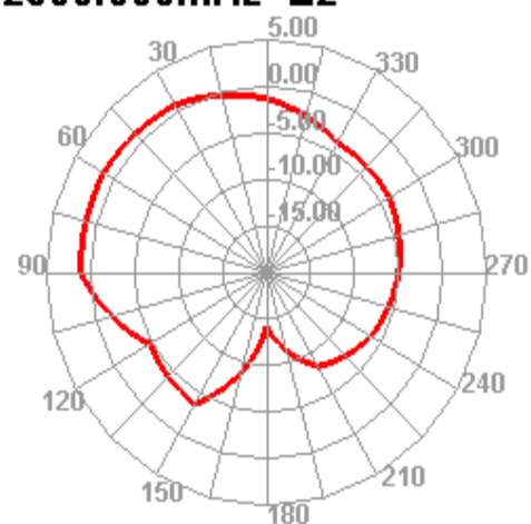
2500.000MHz E2
