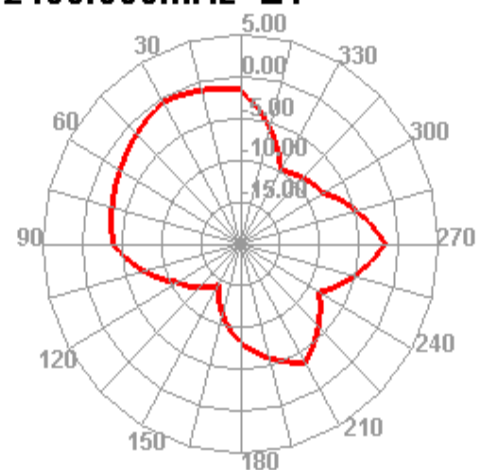
2450.000MHz
