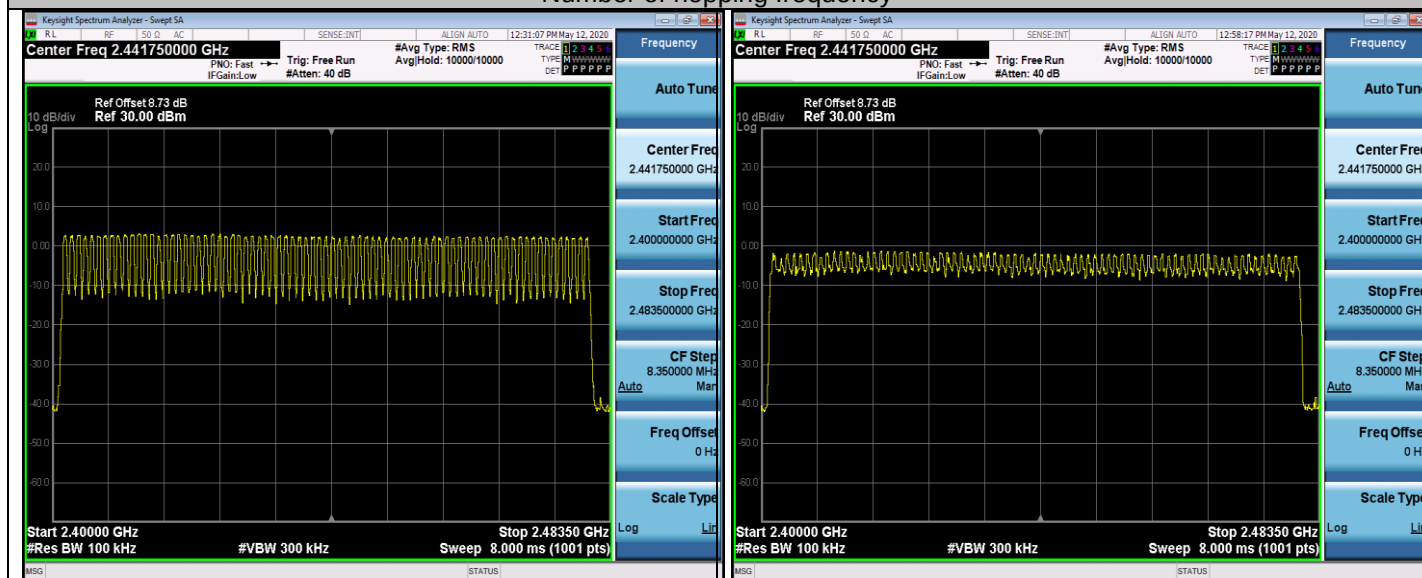
GFSK
