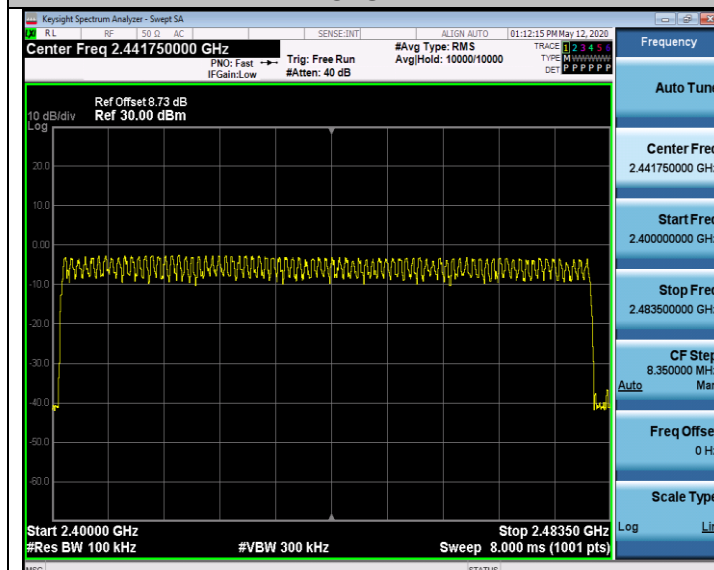
8DPSK
