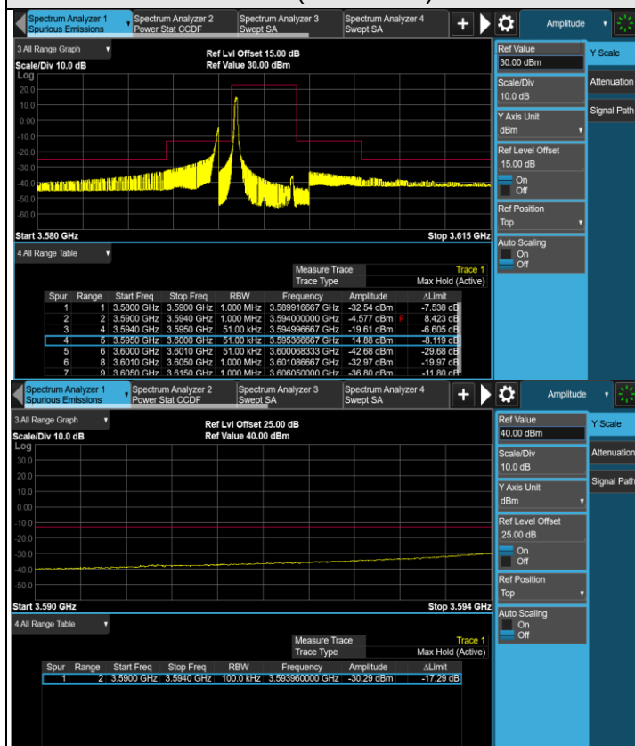
1RB#0 (3597.5MHz)
