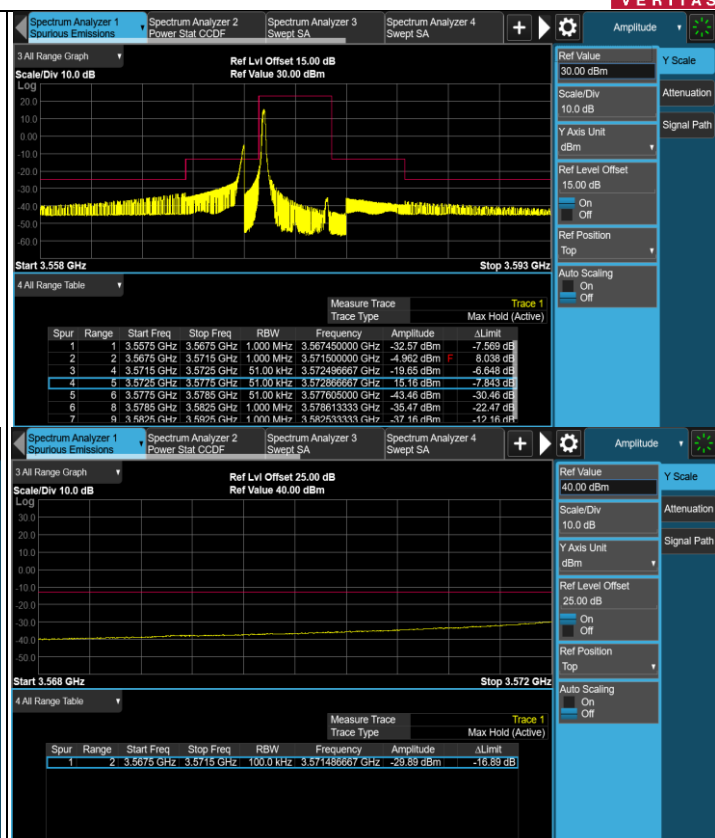
1RB#0 (3575MHz)
