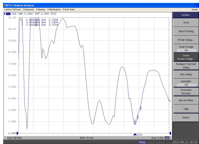
VSWR
