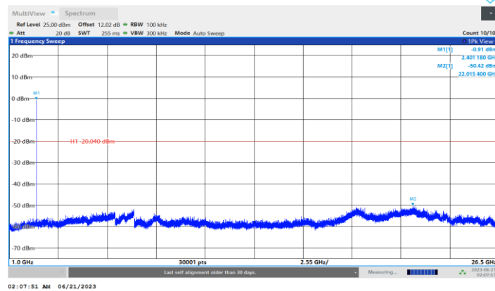
BLE 2M Ant1 2402 1000~26500
