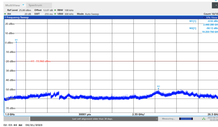
BLE 1M Ant1 2440 1000~26500
