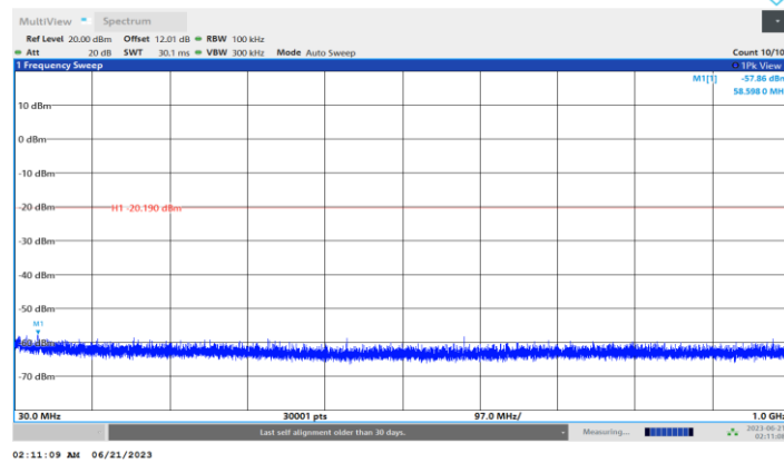
BLE 2M Ant1 2480 30~1000
