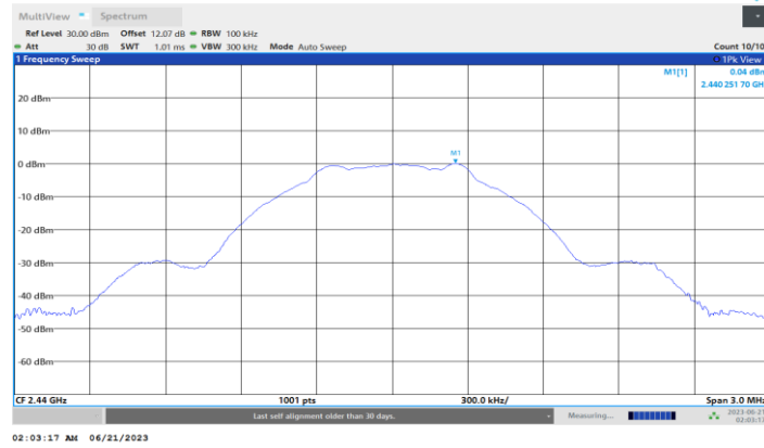
BLE 1M Ant1 2440 0~Reference
