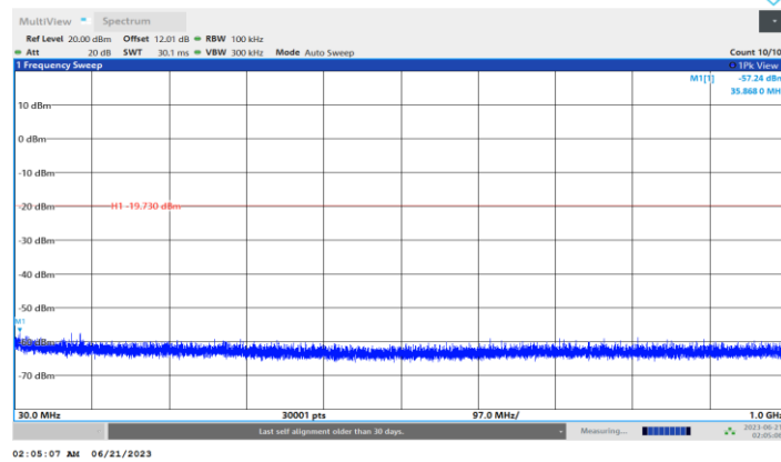
BLE 1M Ant1 2480 30~1000
