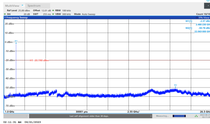
BLE 2M Ant1 2480 1000~26500
