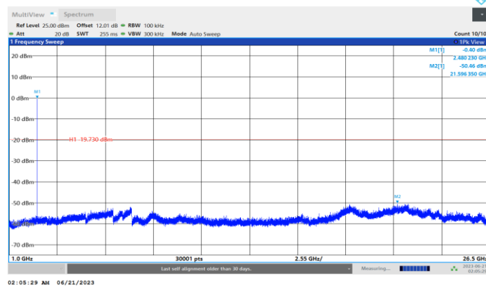
BLE 1M Ant1 2480 1000~26500
