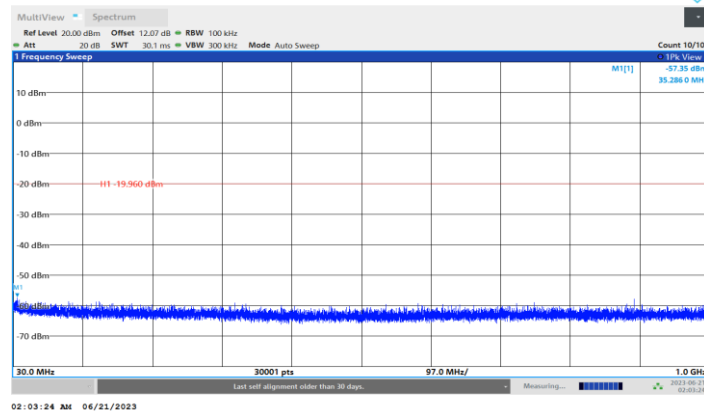
BLE 1M Ant1 2440 30~1000
