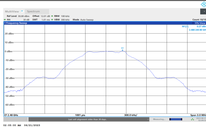
BLE 1M Ant1 2480 0~Reference
