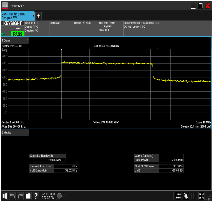
n66_20MHz_15kHz_1745MHz_DFT-s-OFDM PI/2 BPSK_RB106@0
