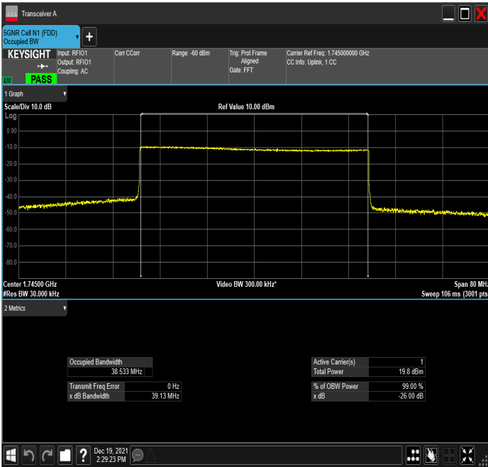
n66_40MHz_15kHz_1745MHz_CP-OFDM QPSK_RB216@0
