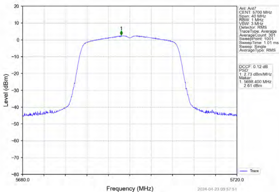
802.11n(HT20)_HCH_5700MHz_Ant7_NTNV
