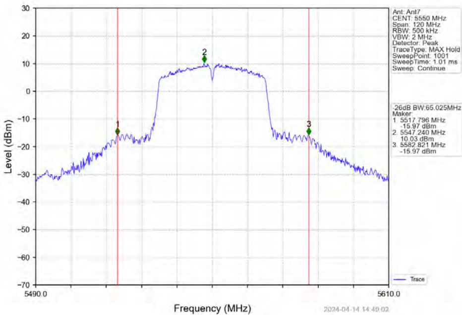
802.11n(HT40) MCH_5550MHz_Ant7_NTNV
