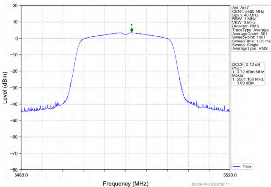
802.11n(HT20)_LCH_5500MHz_Ant7_NTNV
