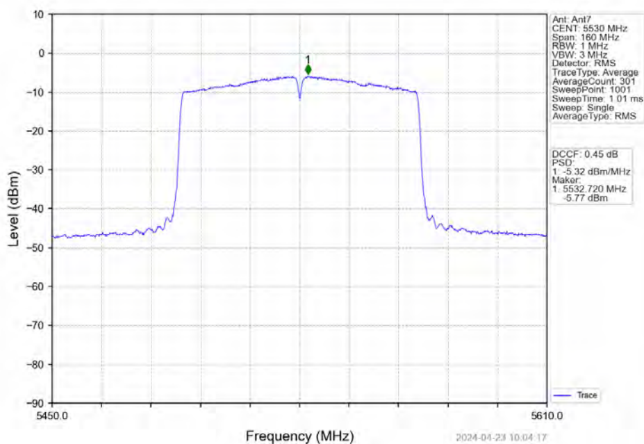
802.11ac(VHT80)_LCH_5530MHz_Ant7_NTNV
