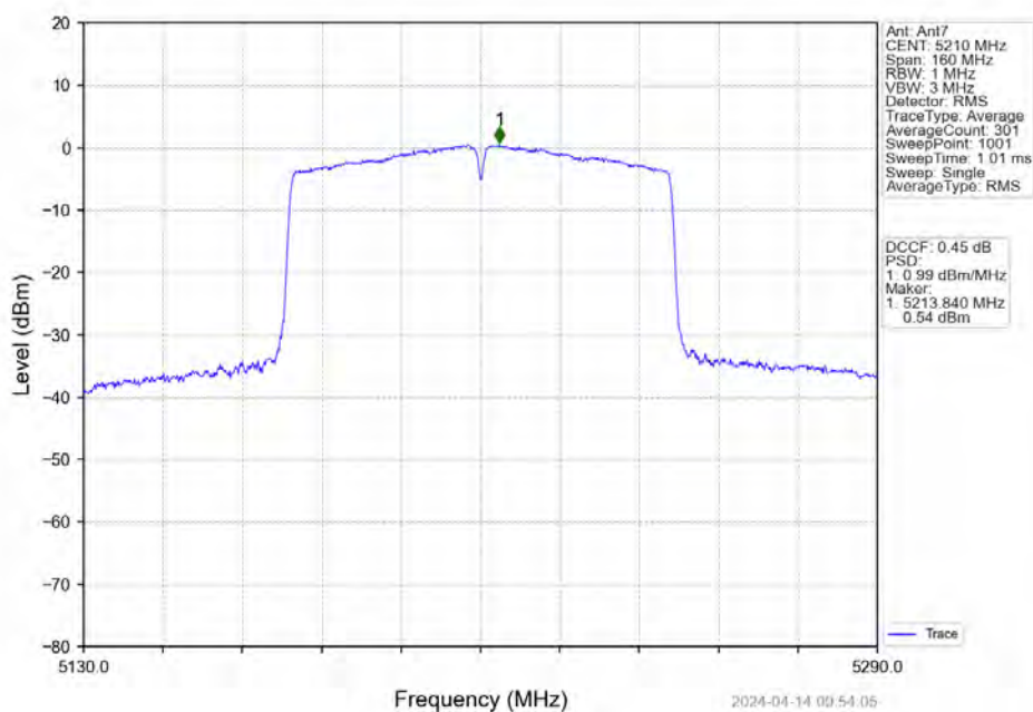
802.11ac(VHT80)_MCH_5210MHz_Ant7_NTNV
