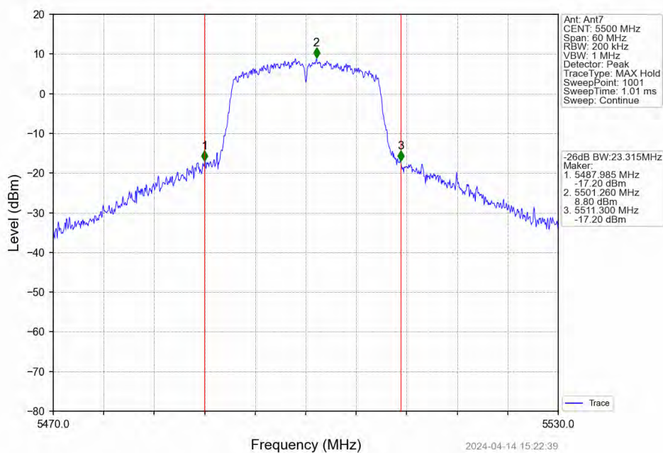
802.11ac(VHT20)_LCH_5500MHz_Ant7_NTNV
