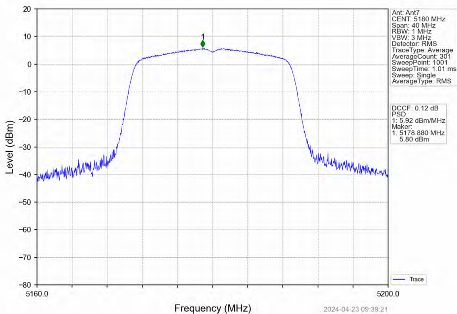
802.11n(HT20)_LCH_5180MHz_Ant7_NTNV
