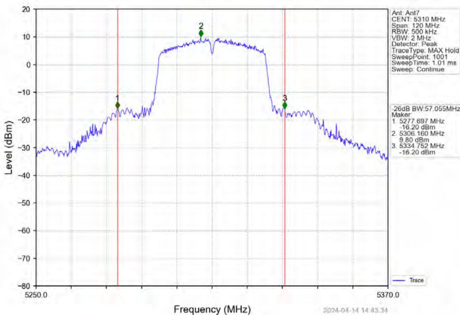
802.11n(HT40) HCH_5310MHz_Ant7_NTNV
