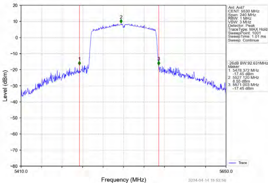
802.11ac(VHT80)_LCH_5530MHz_Ant7_NTNV
