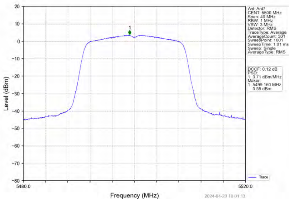
802.11ac(VHT20)_LCH_5500MHz_Ant7_NTNV
