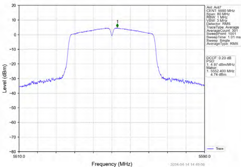
802.11n(HT40) MCH_5550MHz_Ant7_NTNV
