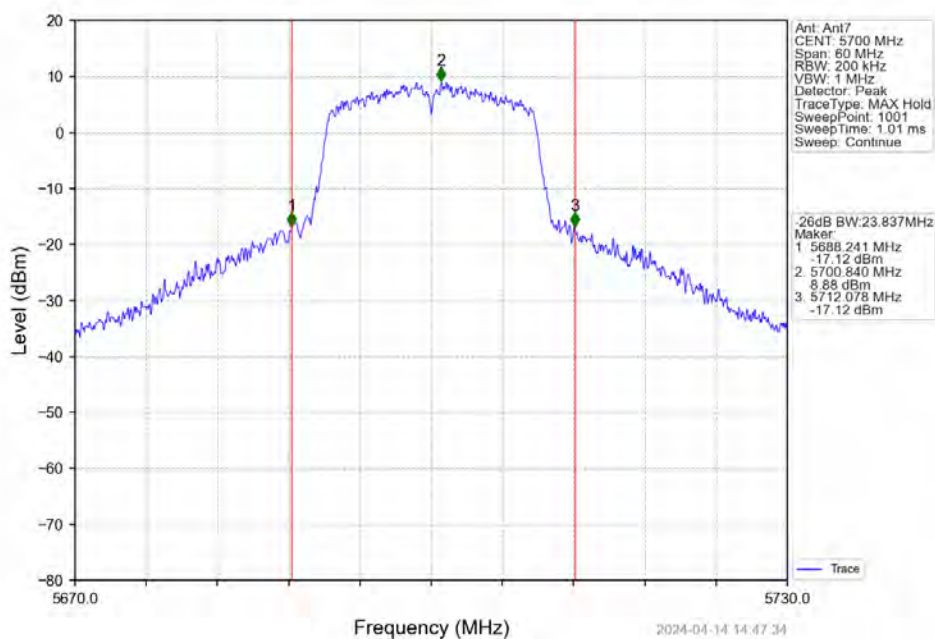
802.11n(HT20)_HCH_5700MHz_Ant7_NTNV
