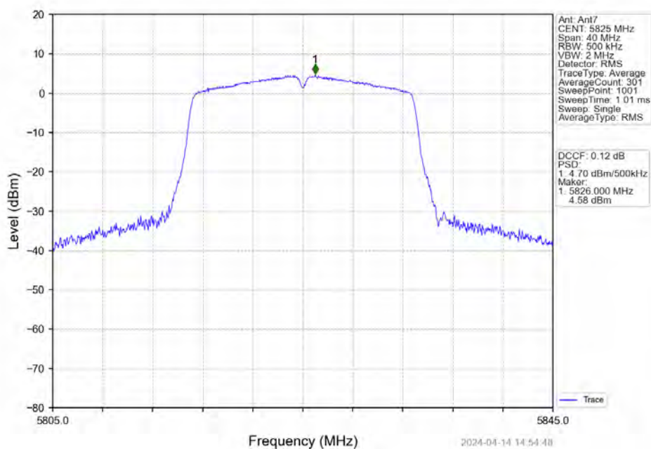
802.11n(HT20)_HCH_5825MHz_Ant7_NTNV
