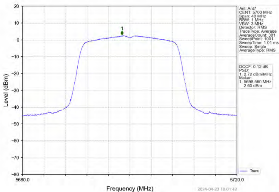
802.11ac(VHT20)_HCH_5700MHz_Ant7_NTNV
