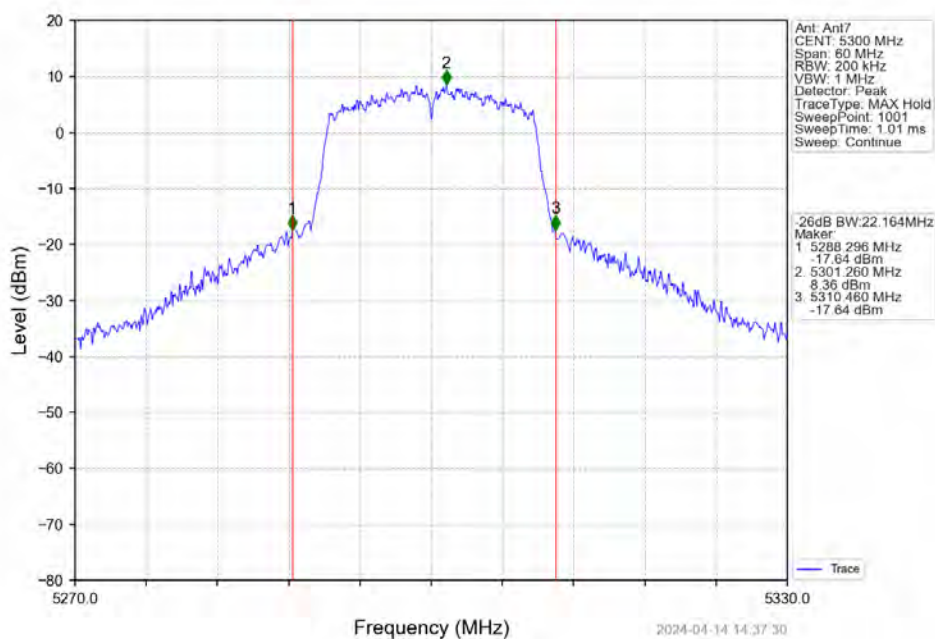
802.11n(HT20) MCH_5300MHz_Ant7_NTNV
