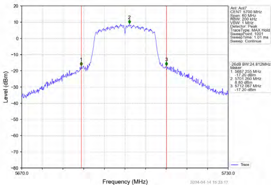
802.11ac(VHT20)_HCH_5700MHz_Ant7_NTNV
