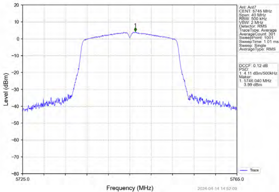
802.11n(HT20)_LCH_5745MHz_Ant7_NTNV
