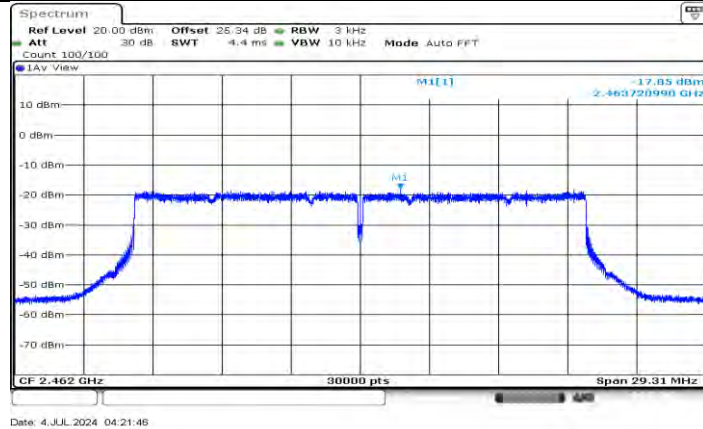
11AX20SISO_Ant1_2462
