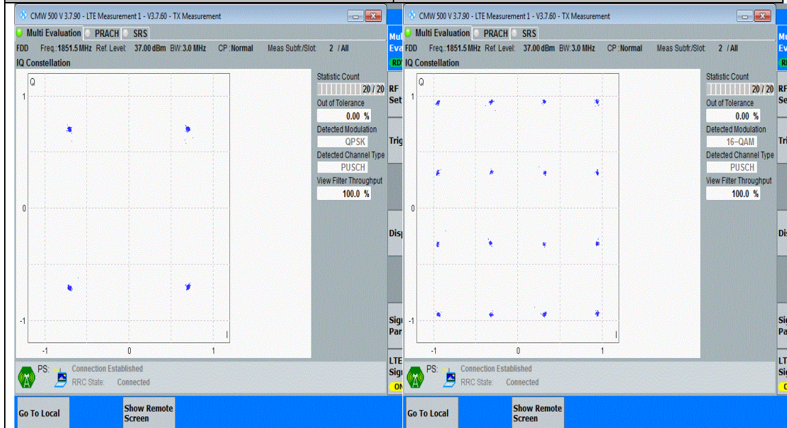
Band2-3MHz-QPSK-18615-15RB#0-PASS
