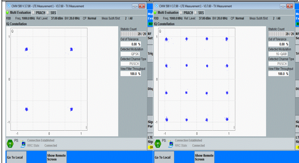
Band2-20MHz-QPSK-18700-100RB#0-PASS
