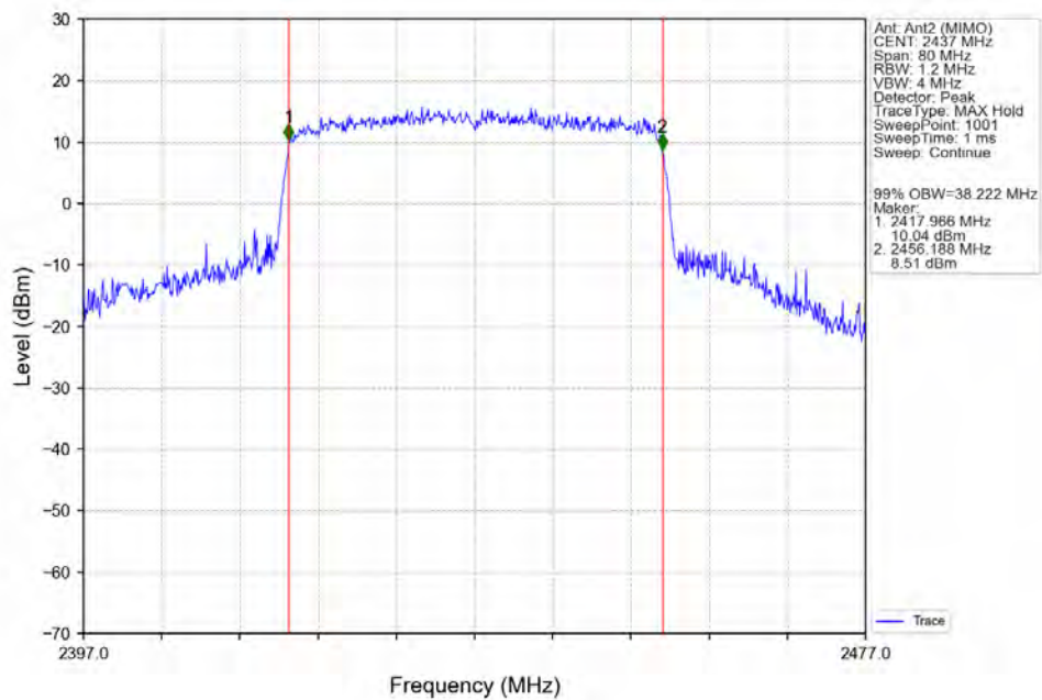
802.11ax(HEW40) MCH 2437MHz RU484 Left Ant2 (MIMO) NTVN
