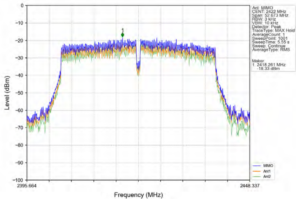
802.11n(HT40)_LCH_2422MHz MIMO NTV
