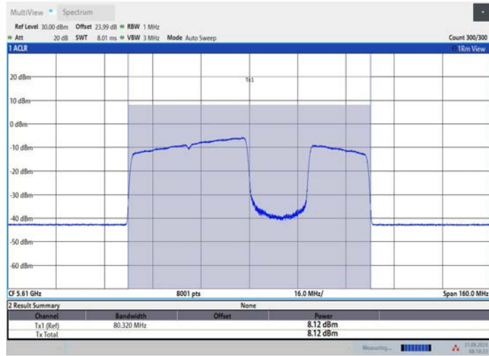
11BE80MIMO_Ant3_5610_484+242_OFDMA_3
