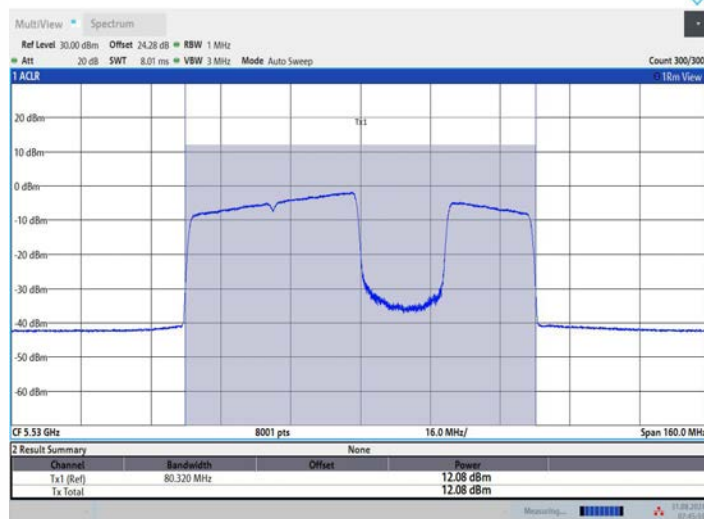
11BE80MIMO_Ant1_5530_484+242_OFDMA_4
