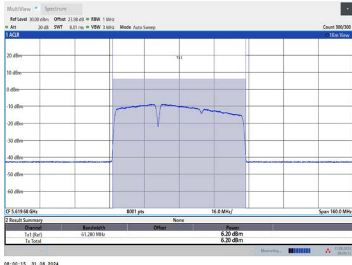
11BE80MIMO_Ant2_5610_484+242_OFDMA_1
