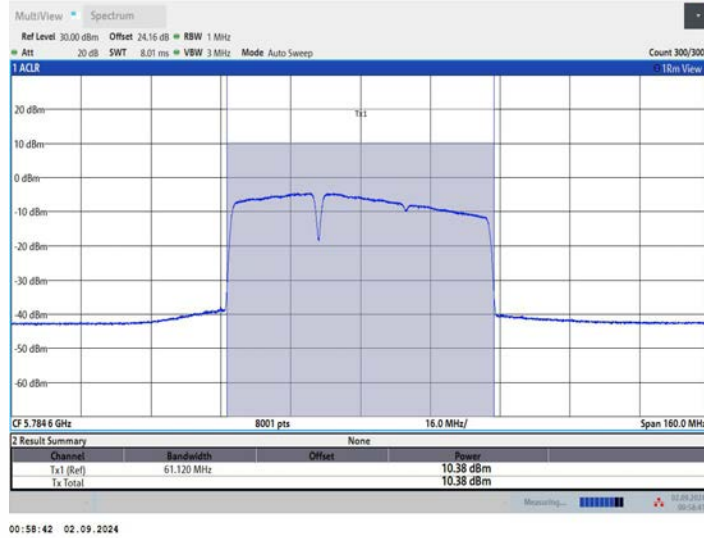
11BE80MIMO_Ant3_5775_484+242_OFDMA_2
