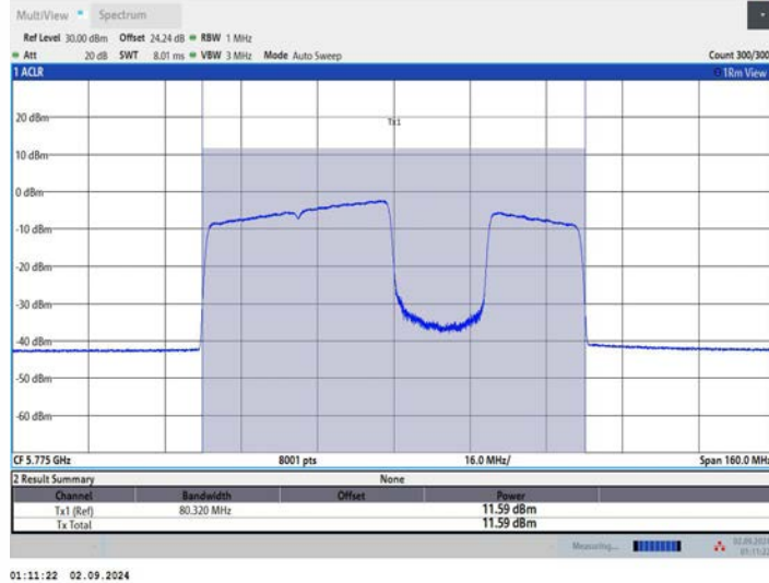
11BE80MIMO_Ant1_5775_484+242_OFDMA_4
