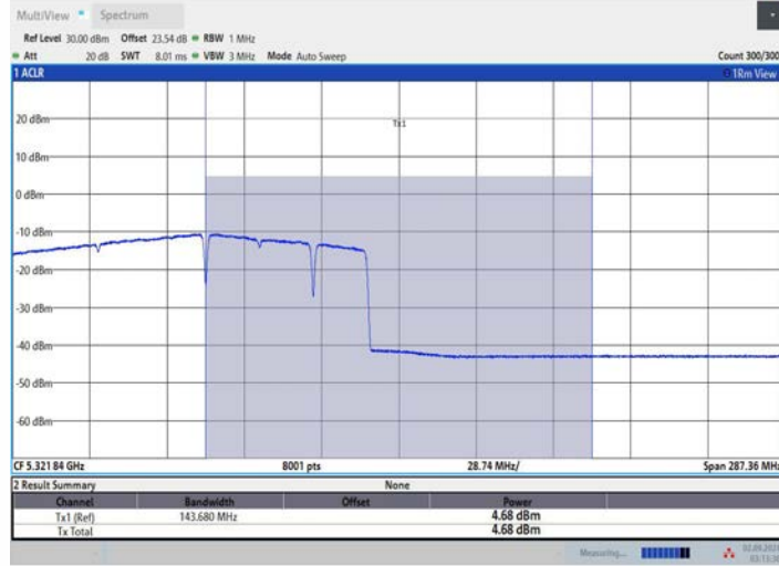
11BE160MIMO_Ant3 5250 UNII-2A 996+484+242 OFDMA 8
