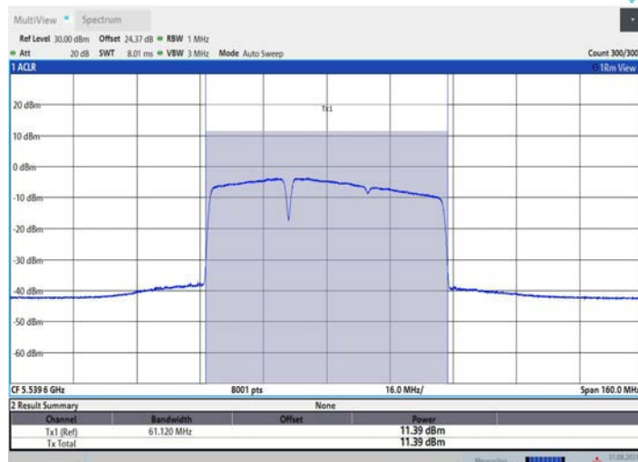
11BE80MIMO_Ant2_5530_484+242_OFDMA_2
