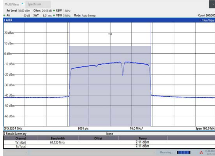
11BE80MIMO_Ant2_5530_484+242_OFDMA_4
