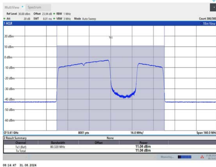
11BE80MIMO_Ant2_5610_484+242_OFDMA_4
