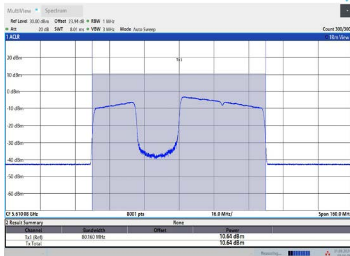
11BE80MIMO_Ant2_5610_484+242_OFDMA_3
