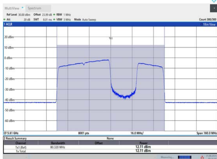
11BE80MIMO_Ant3_5610_484+242_OFDMA_4
