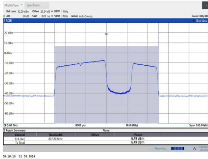
11BE80MIMO_Ant2_5610_484+242_OFDMA_3
