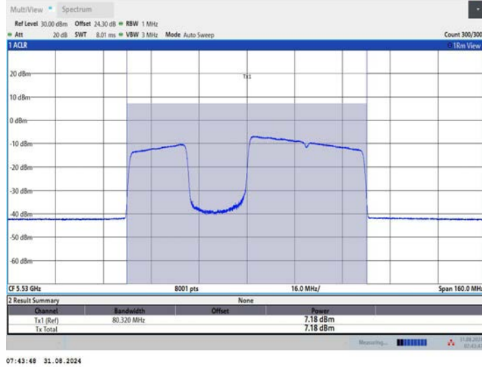
11BE80MIMO_Ant3_5530_484+242_OFDMA_2
