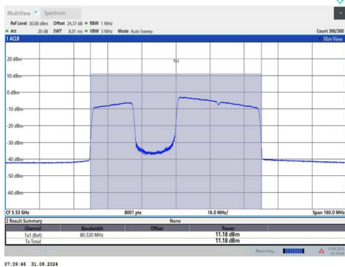
11BE80MIMO_Ant2_5530_484+242_OFDMA_3
