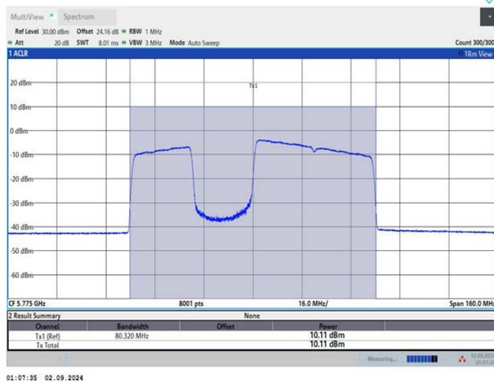
11BE80MIMO_Ant3_5775_484+242_OFDMA_3
