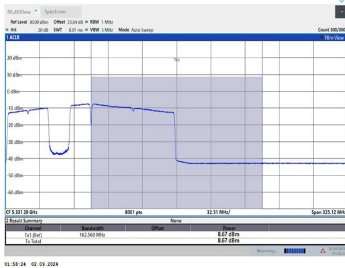
11BE160MIMO_Ant2_5250_UNII-2A_996+484+242_OFDMA_4
