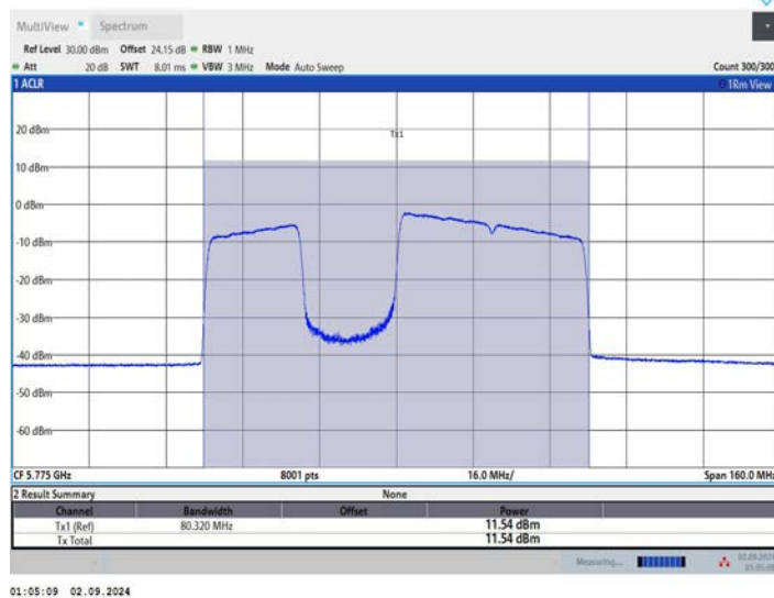
11BE80MIMO_Ant2_5775_484+242_OFDMA_3
