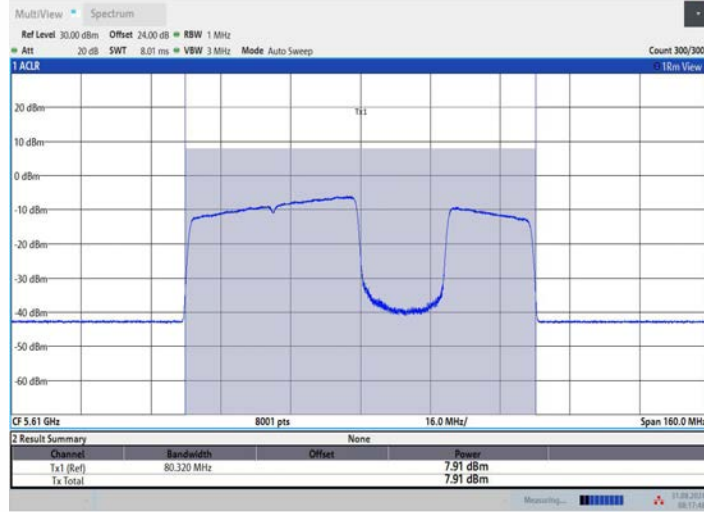
11BE80MIMO_Ant1_5610_484+242_OFDMA_3
