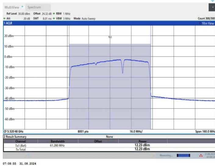
11BE80MIMO_Ant2_5530_484+242_OFDMA_1
