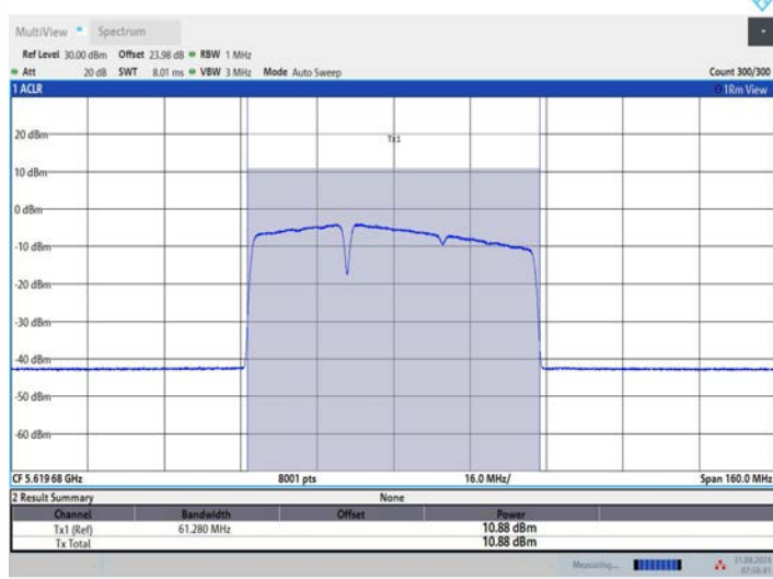
11BE80MIMO_Ant2_5610_484+242_OFDMA_2
