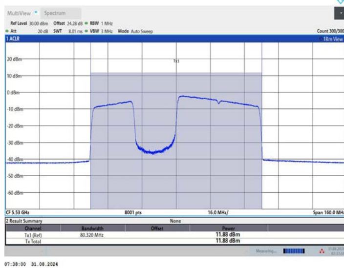
11BE80MIMO_Ant1_5530_484+242_OFDMA_3
