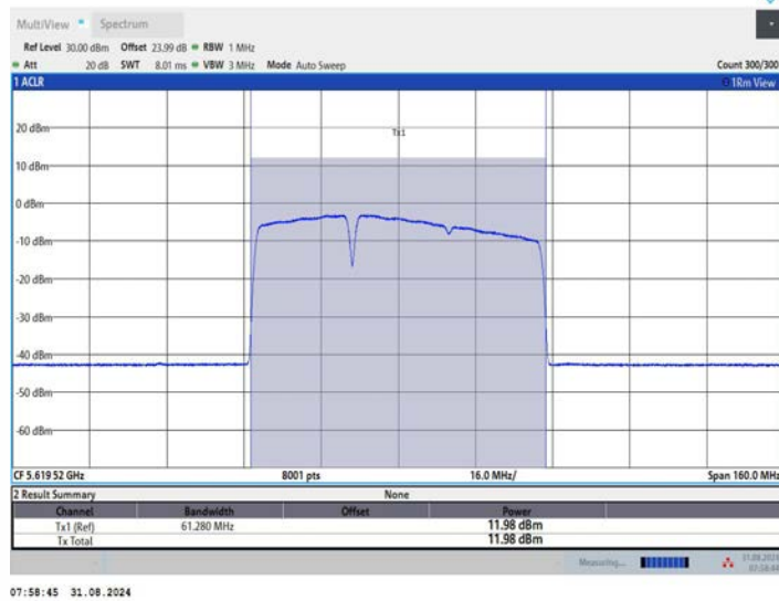
11BE80MIMO_Ant3_5610_484+242_OFDMA_2
