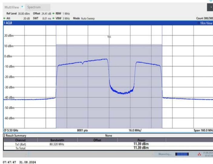
11BE80MIMO_Ant2_5530_484+242_OFDMA_4
