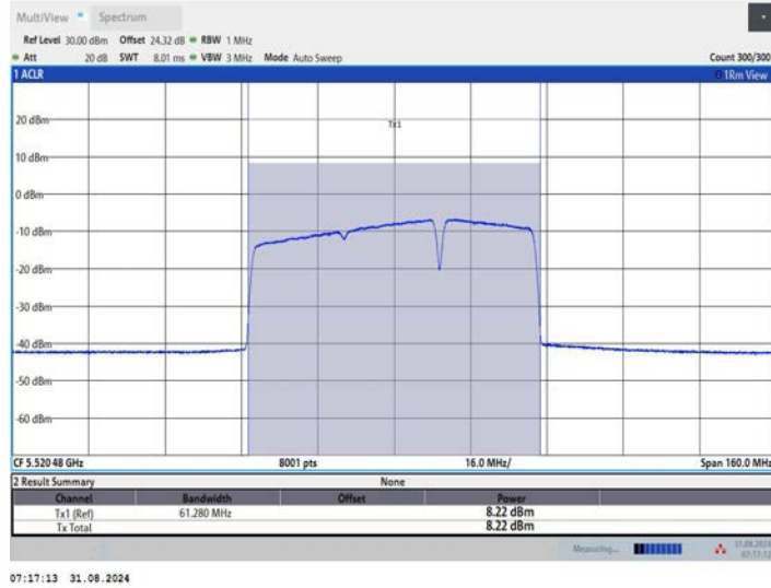
11BE80MIMO_Ant1_5530_484+242_OFDMA_4
