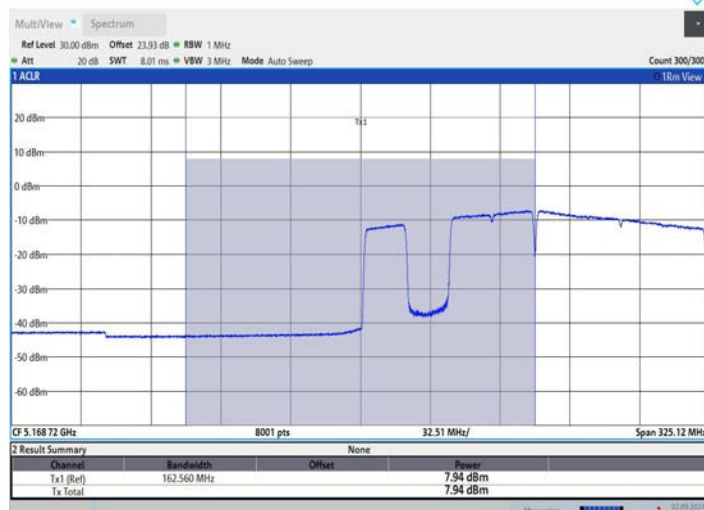
11BE160MIMO_Ant2_5250_UNII-1_996+484+242_OFDMA_3
