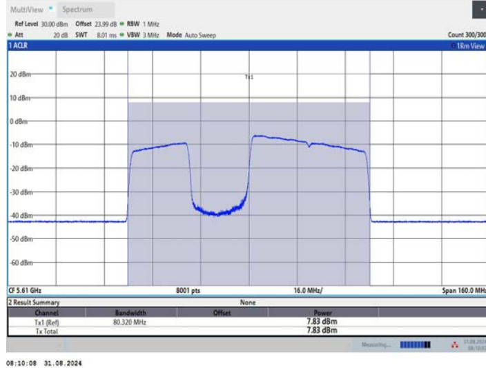
11BE80MIMO_Ant3_5610_484+242_OFDMA_2
