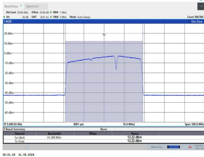
11BE80MIMO_Ant2_5610_484+242_OFDMA_1
