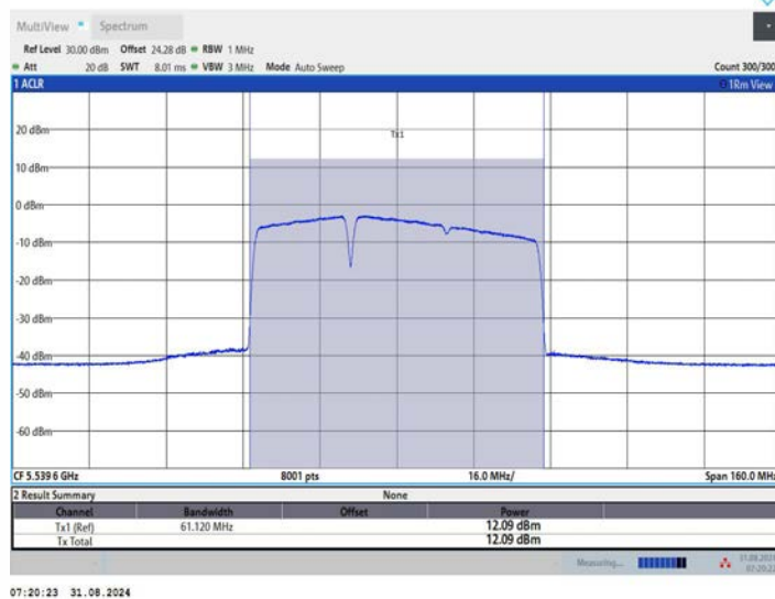
11BE80MIMO_Ant1_5530_484+242_OFDMA_2
