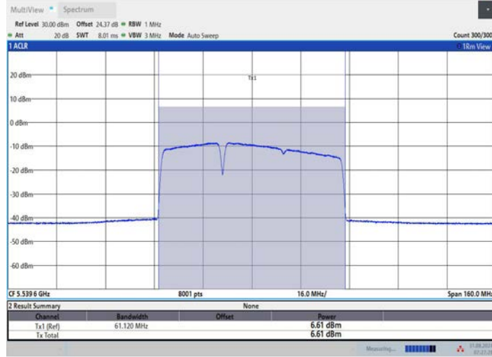
11BE80MIMO_Ant2_5530_484+242_OFDMA_1
