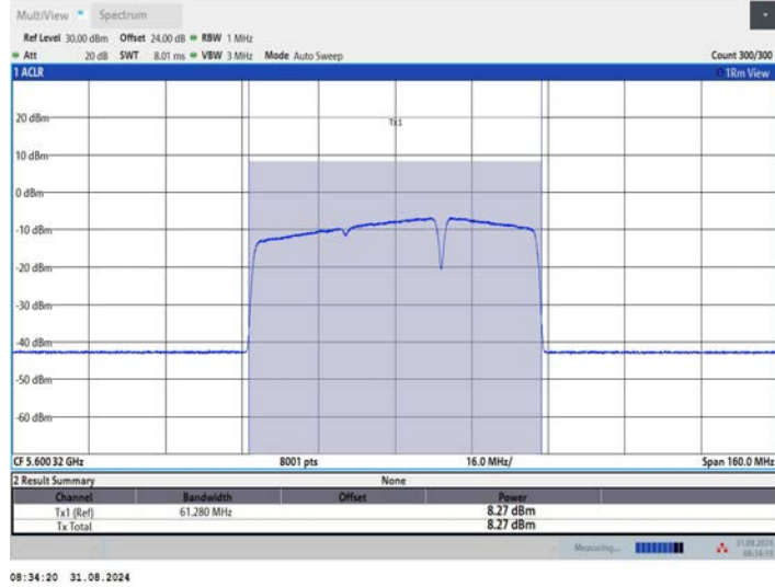
11BE80MIMO_Ant1_5610_484+242_OFDMA_4
