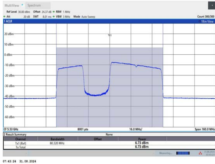
11BE80MIMO_Ant2_5530_484+242_OFDMA_2
