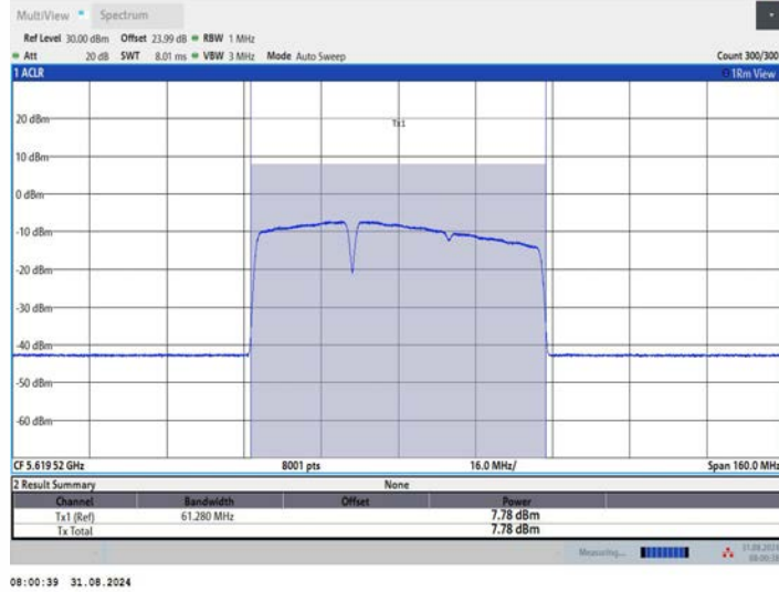
11BE80MIMO_Ant3_5610_484+242_OFDMA_1
