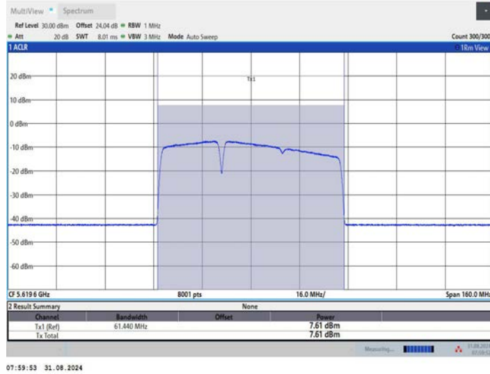
11BE80MIMO_Ant1_5610_484+242_OFDMA_1
