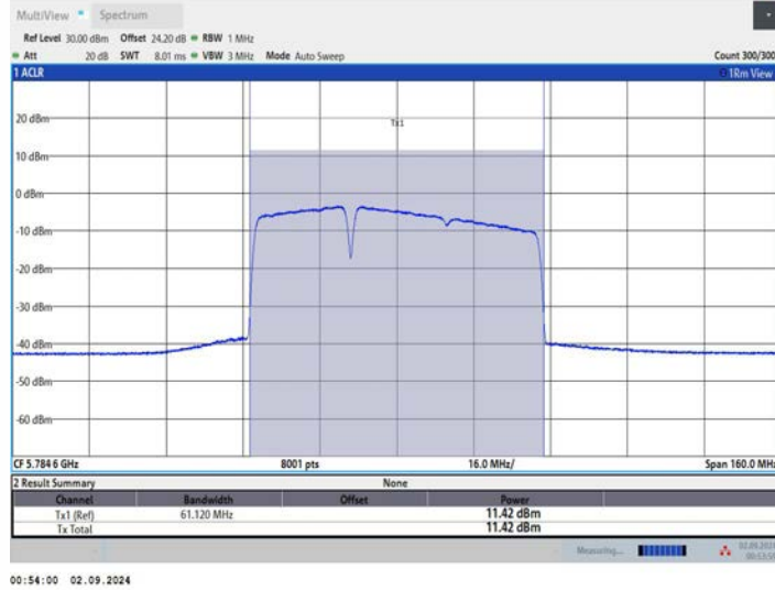
11BE80MIMO_Ant1_5775_484+242_OFDMA_2
