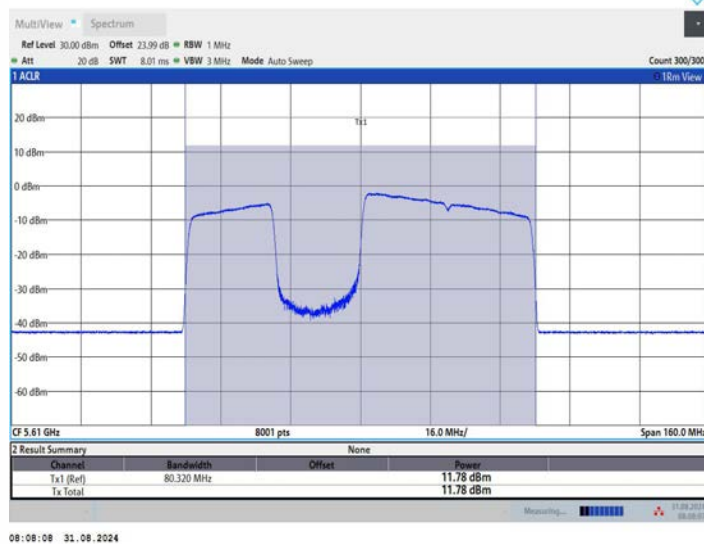
11BE80MIMO_Ant3_5610_484+242_OFDMA_3
