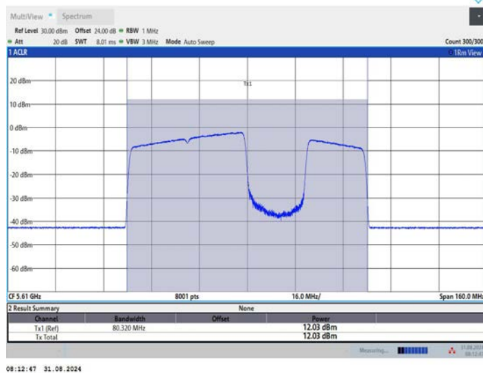
11BE80MIMO_Ant1_5610_484+242_OFDMA_4
