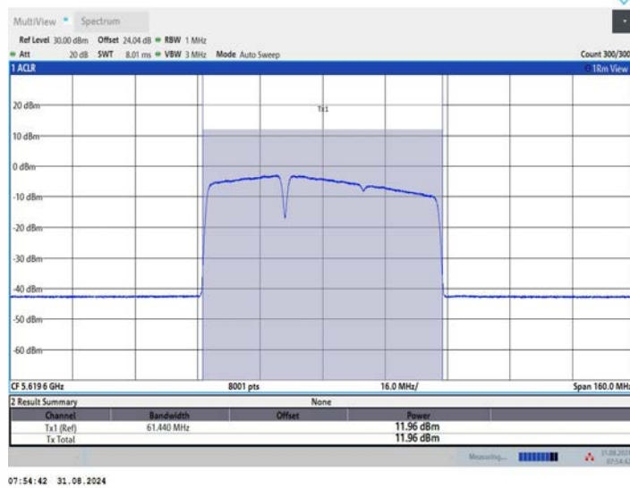
11BE80MIMO_Ant1_5610_484+242_OFDMA_2
