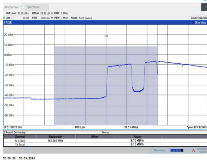
11BE160MIMO_Ant3_5250_UNII-1_996+484+242_OFDMA_4
