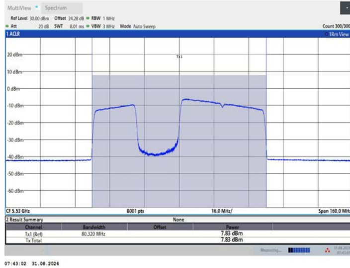
11BE80MIMO_Ant1_5530_484+242_OFDMA_2
