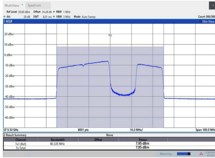
11BE80MIMO_Ant1_5530_484+242_OFDMA_3
