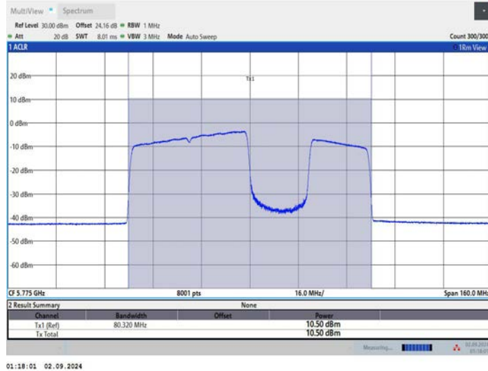
11BE80MIMO_Ant3_5775_484+242_OFDMA_4
