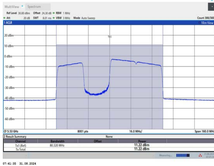
11BE80MIMO_Ant3_5530_484+242_OFDMA_3
