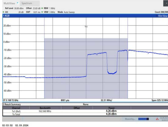
11BE160MIMO_Ant3_5250_UNII-1_996+484+242_OFDMA_3
