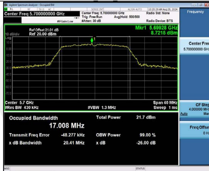
11A_Ant2_5700
