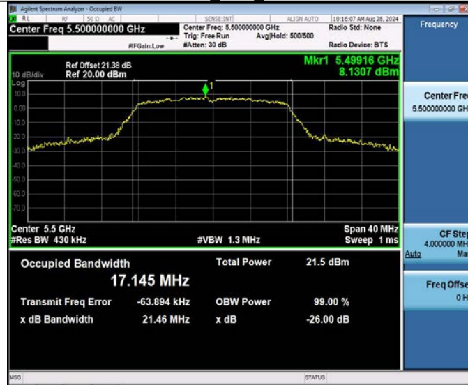
11A_Ant2_5500
