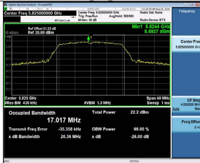
11A_Ant2_5825
