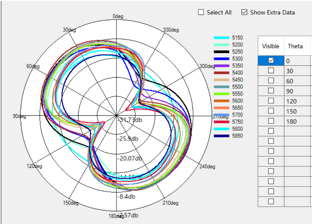
5G Phi=0deg
