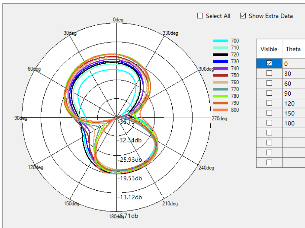
LTEB12/B17/B28 Phi=0deg
