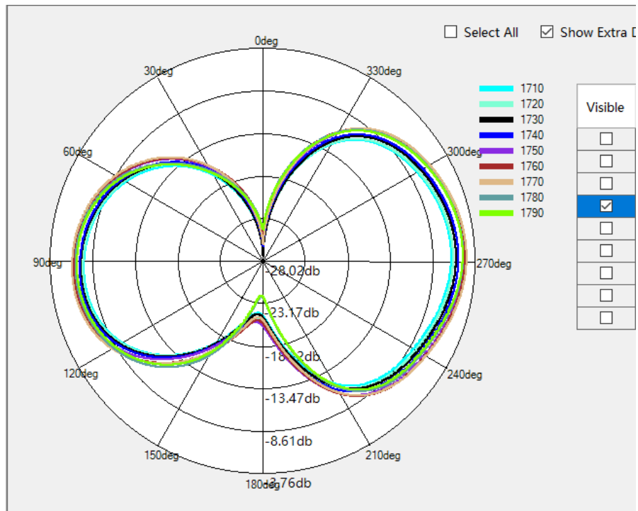
LTE B3 B4 B66 G1800 W4 Phi=90deg
