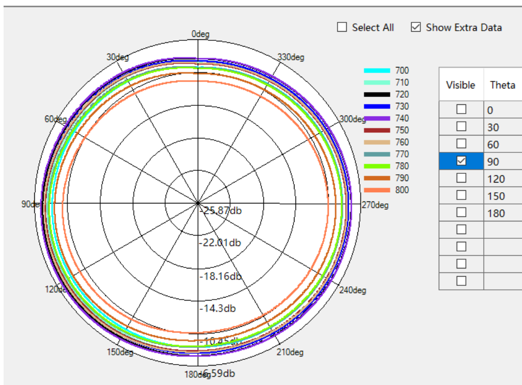
LTEB12/B17/B28 Theta=90deg
