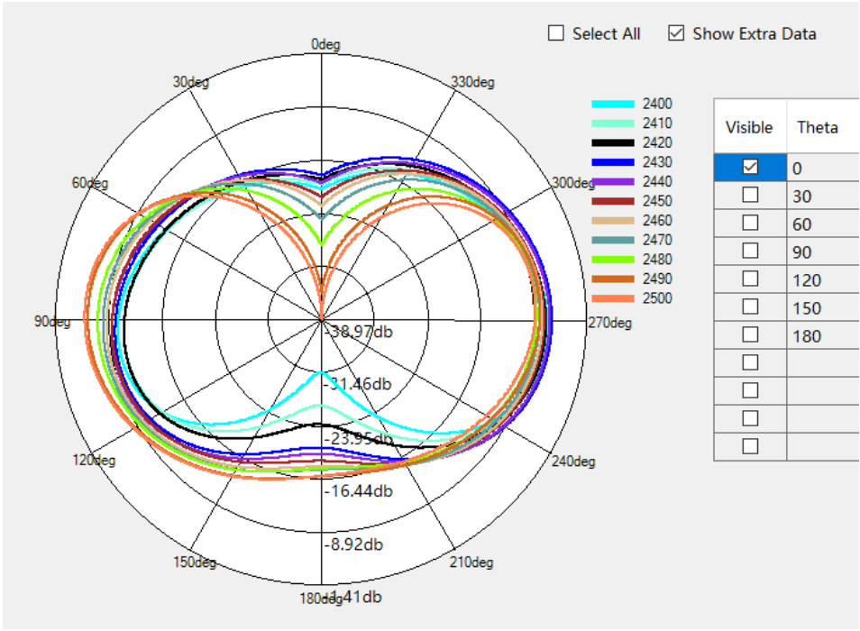
2.4G/BT Phi=0deg
