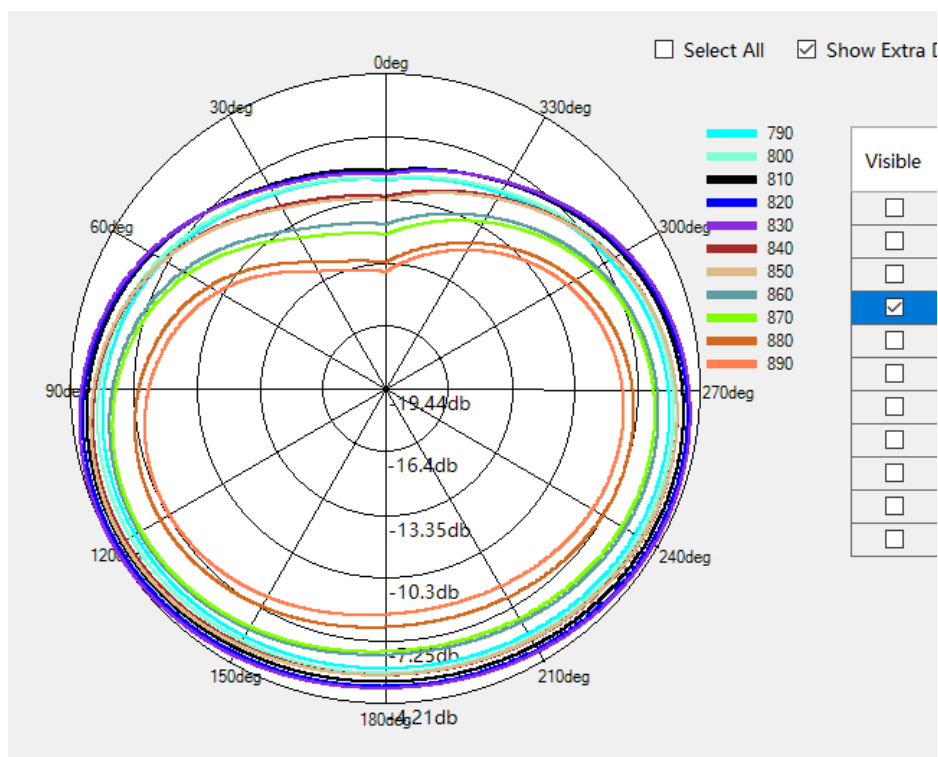
GSM850/WCDMA B5/ LTE B5/B20 Theta=90deg
