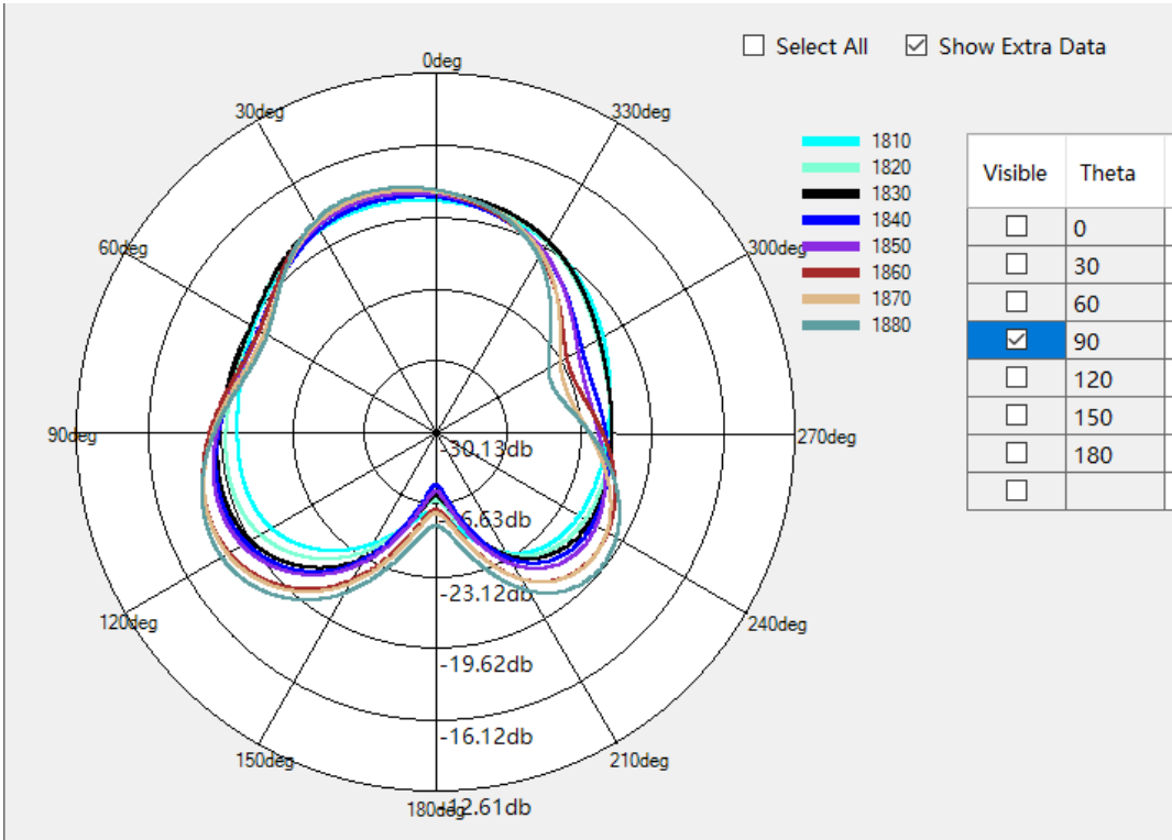
B3 Theta=90deg
