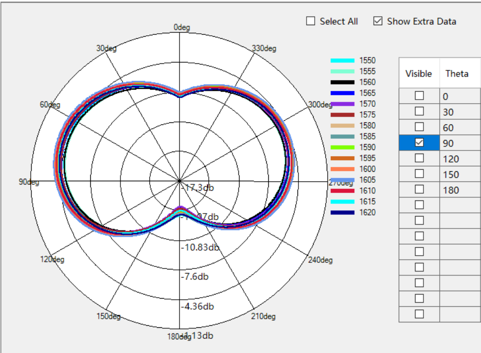
GPS Theta=90deg
