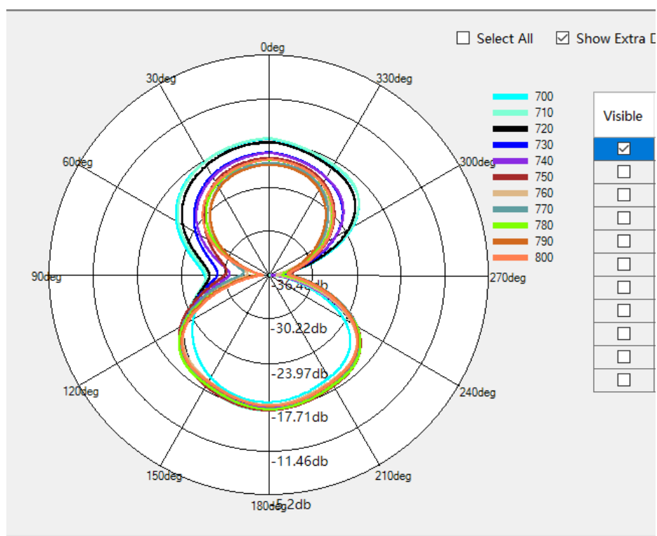
LTEB12/B17/B28 Phi=0deg
