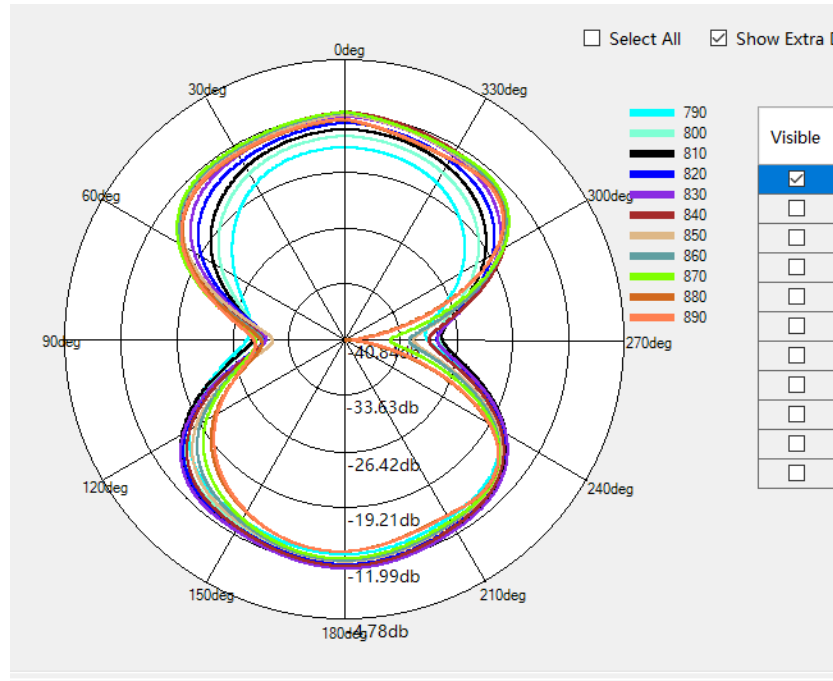
GSM850/WCDMA B5/ LTE B5/B20 Phi=0deg
