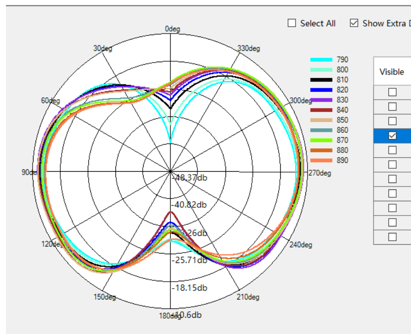
GSM850/WCDMA B5/ LTE B5/B20 Phi=90deg
