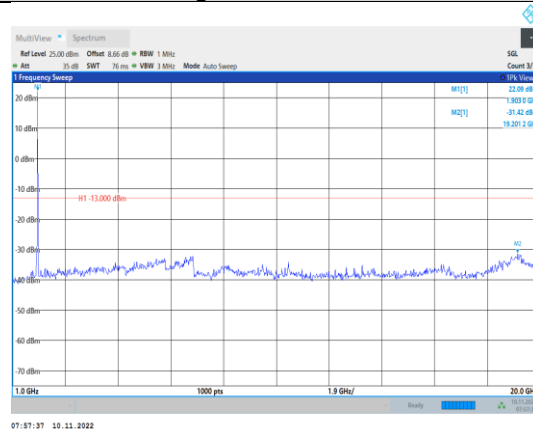
Band2-15MHz-QPSK-19125-1RB#0- Range2:1000~20000MHz
