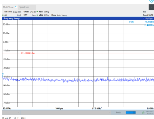
Band4-3MHz-QPSK-19965-1RB#0- Range1:30~1000MHz
