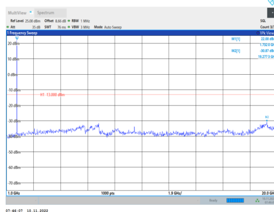
Band4-3MHz-QPSK-20175-1RB#0- Range2:1000~20000MHz
