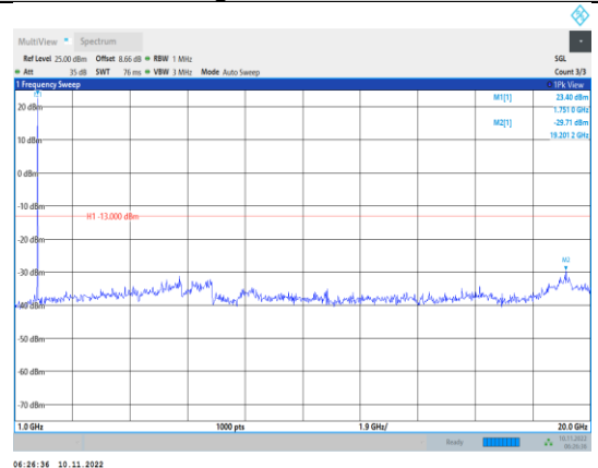
Band4-1.4MHz-QPSK-20393-1RB#0- Range2:1000~20000MHz
