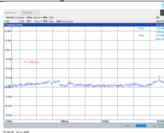
Band2-10MHz-QPSK-19150-1RB#0- Range2:1000~20000MHz
