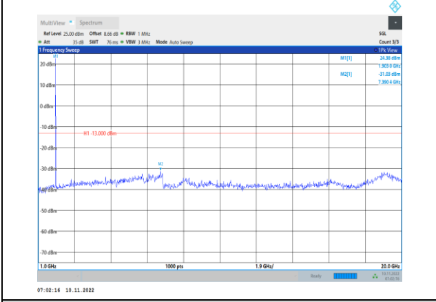
Band2-1.4MHz-QPSK-19193-1RB#0-Range2:1000~20000MHz
