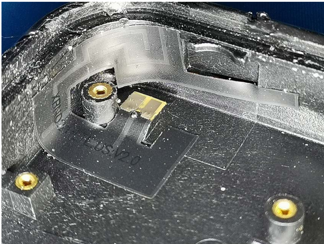
Wi-Fi/BT Antenna
