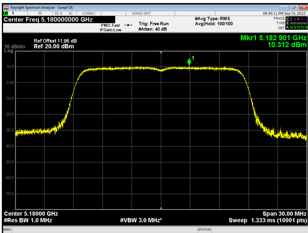
PSD 802.11a 5180MHz Ant1
