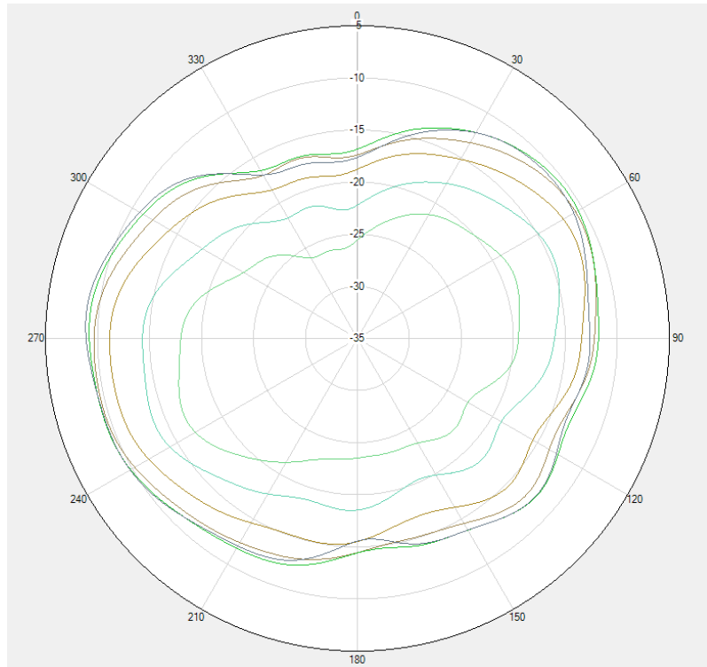
DCS /WCDMA B4/LTE B3/B4/B66 NR n3/n66 Theta=90deg
