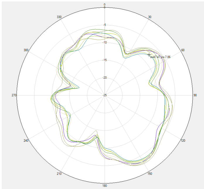
GSM900,B8,N8,WB8 Theta=90deg
