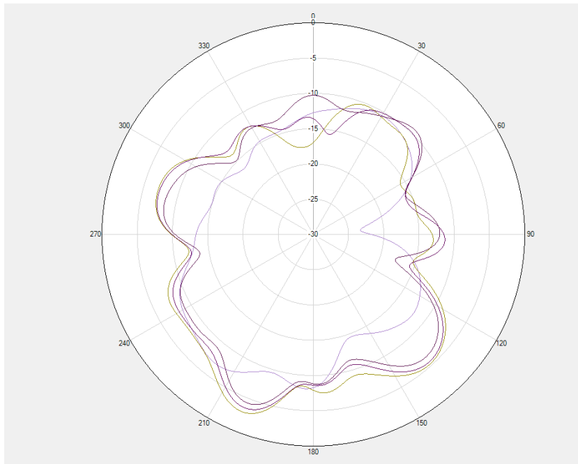
BT/Wifi 2.4G Phi=90deg
