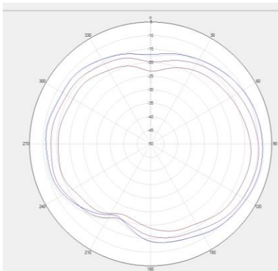
DCS /WCDMA B4/LTE B3/B4/B66 Theta=0deg
