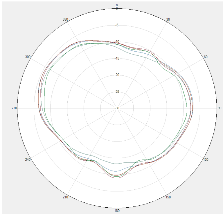
DCS /WCDMA B4/LTE B3/B4/B66 NR n3/n66 \Phi=90^\circ
