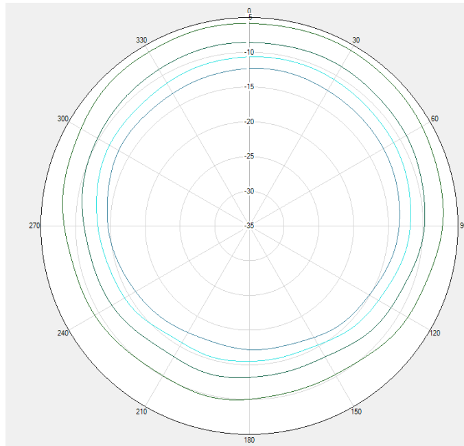
DCS /WCDMA B4/LTE B3/B4/B66 Phi=0deg
