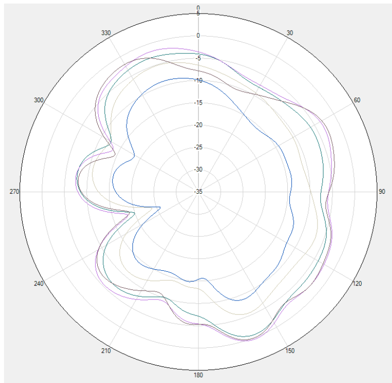
LTE B1/NR n1 \Phi=90^\circ
