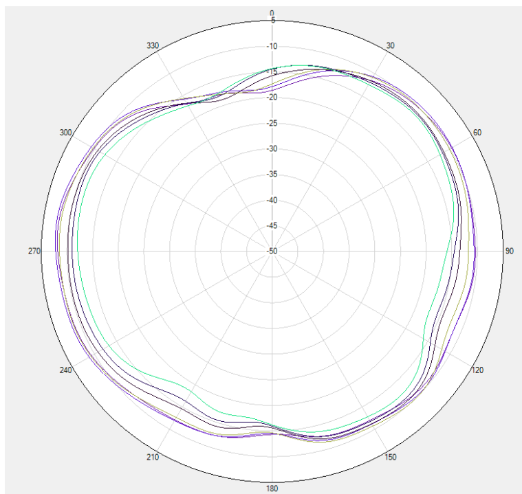
DCS /WCDMA B4/LTE B3/B4/B66 NR n3/n66 Theta=90deg
