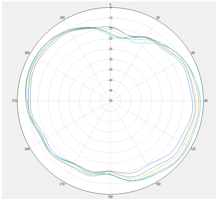
DCS /WCDMA B4/LTE B3/B4/B66 NR n3/n66 Phi=90deg
