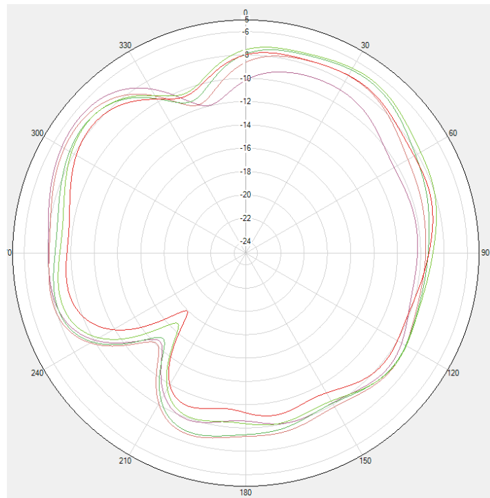
LTE B1/NR n1 Theta=90deg
