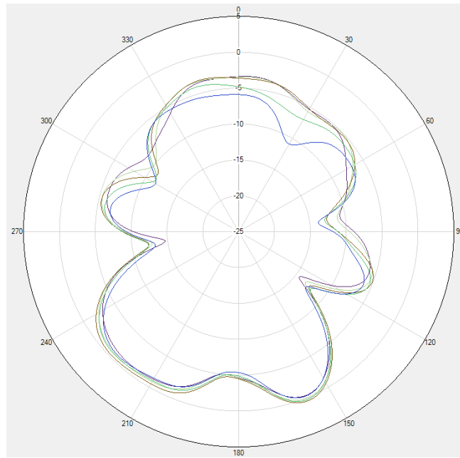
LTE B7/B38/B40/41 NR n7/n38/n40/n41 Theta=90deg
