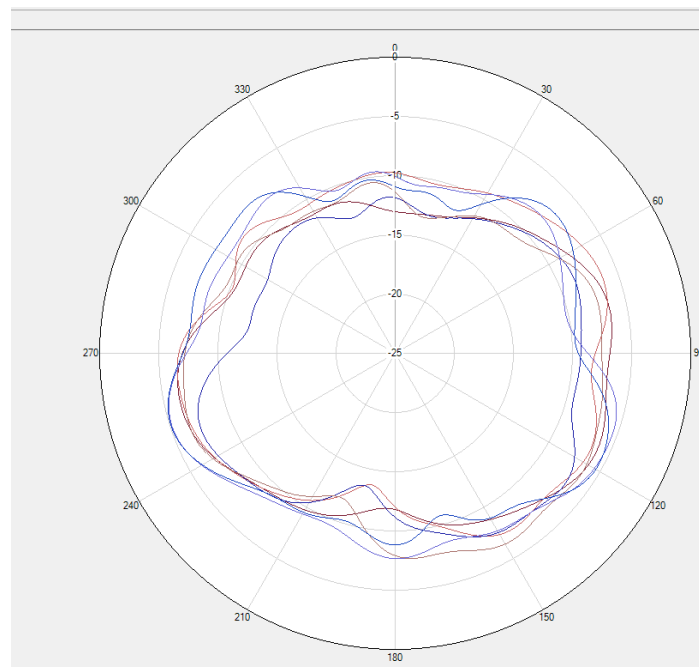
B42/N77/N78 Phi=0deg
