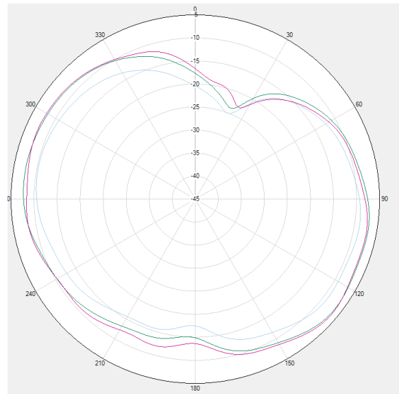
DCS /WCDMA B4/LTE B3/B4/B66 \Theta=90\text{deg}
