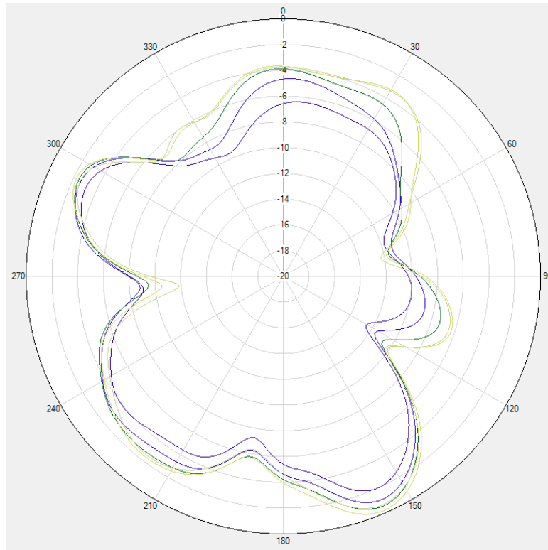
LTE B40/NR n40 Phi=90deg
