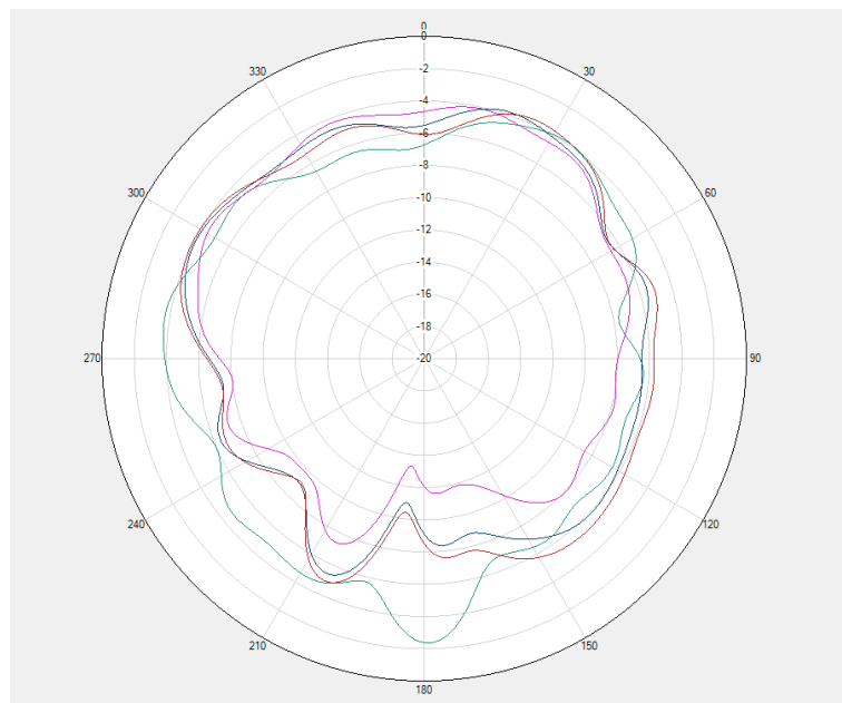
GPS/BT/Wifi 2.4G \Theta=90\text{deg}
