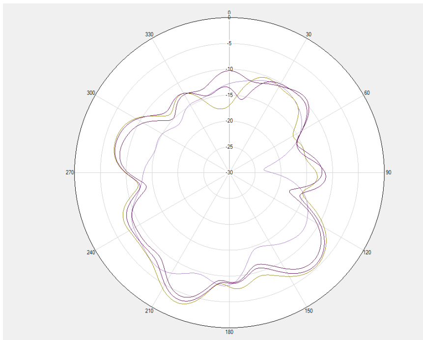
BT/Wifi 2.4G Thera=90deg
