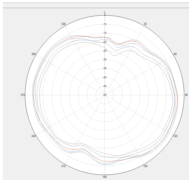
DCS /WCDMA B4/LTE B3/B4/B66 \Theta=90^\circ
