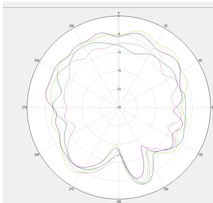
B42/N77/N78 Theta=90deg
