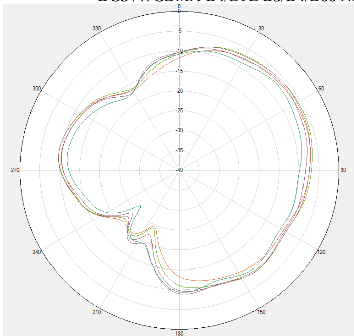
DCS /WCDMA B4/LTE B3/B4/B66 NR n3/n66 \Theta=90^\circ
