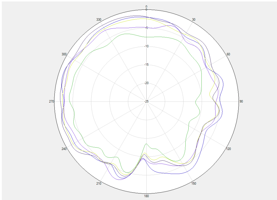
B42/N77/N78 Theta=90deg
