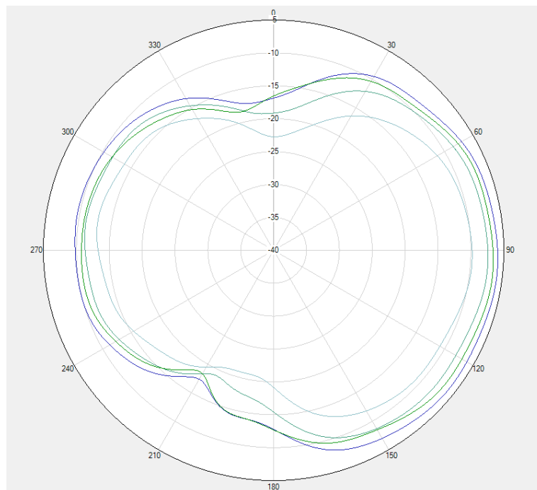
DCS /WCDMA B4/LTE B3/B4/B66 \Phi=90^\circ
