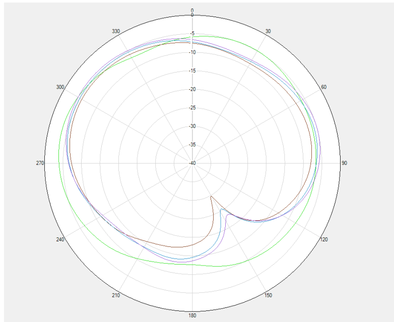
GPS/BT/Wifi 2.4G Phi=0deg
