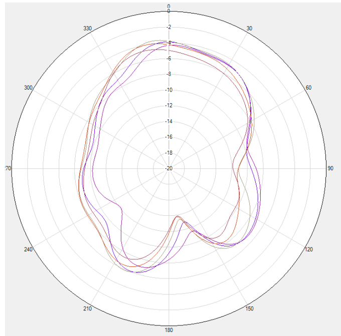
LTE B7/B38/B40/41 NR n7/n38/n40/n41 \Phi=0^\circ
