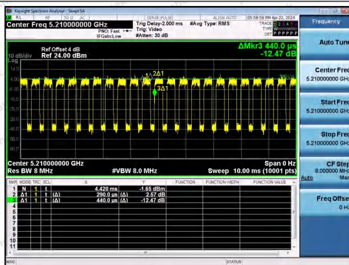
NTNV-11AX80MIMO-Ant1-5210
