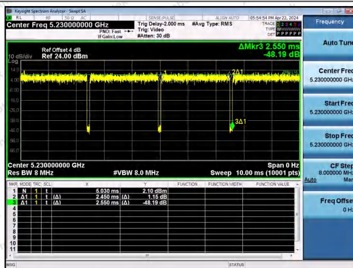
NTNV-11AX40MIMO-Ant1-5230
