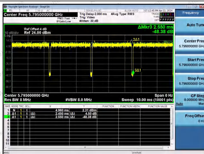
NTNV-11AX40MIMO-Ant2-5795
