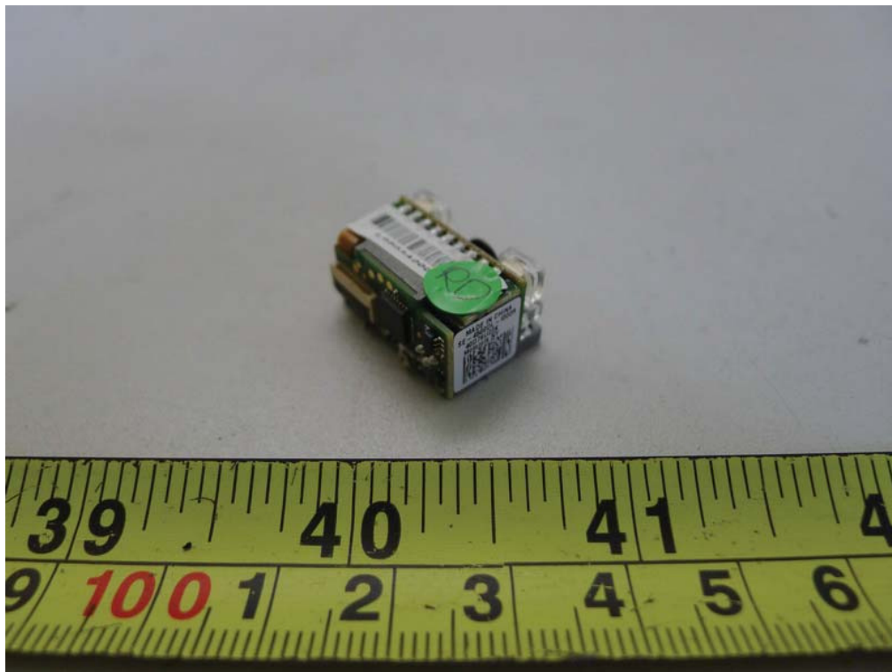
Reader: SE-4500
