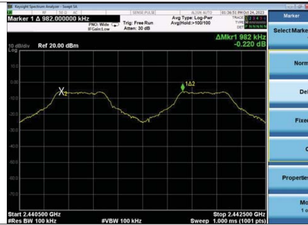
GFSK
