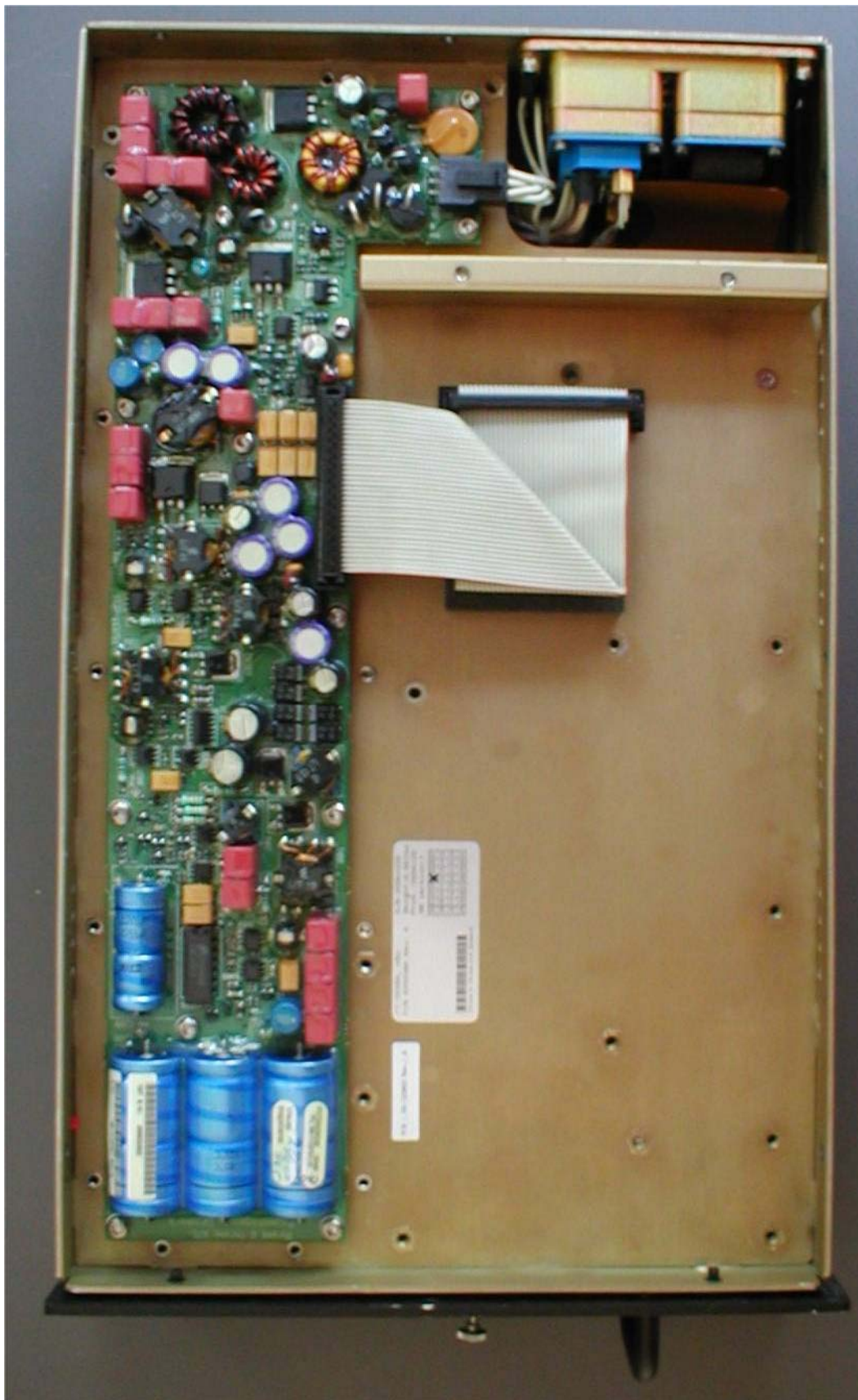
TT93-113751 – Top Side
