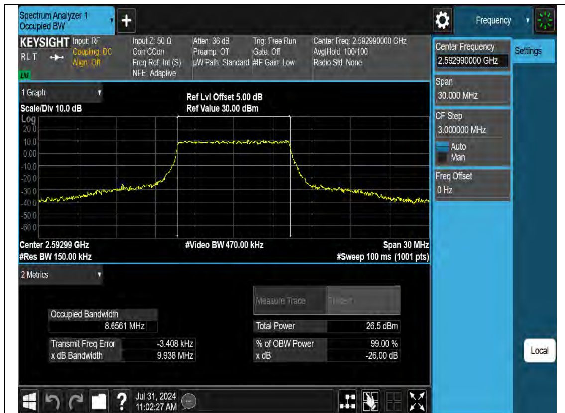
N41-10M-OBW-H-DFT-s-OFDM-Pi2 BPSK
