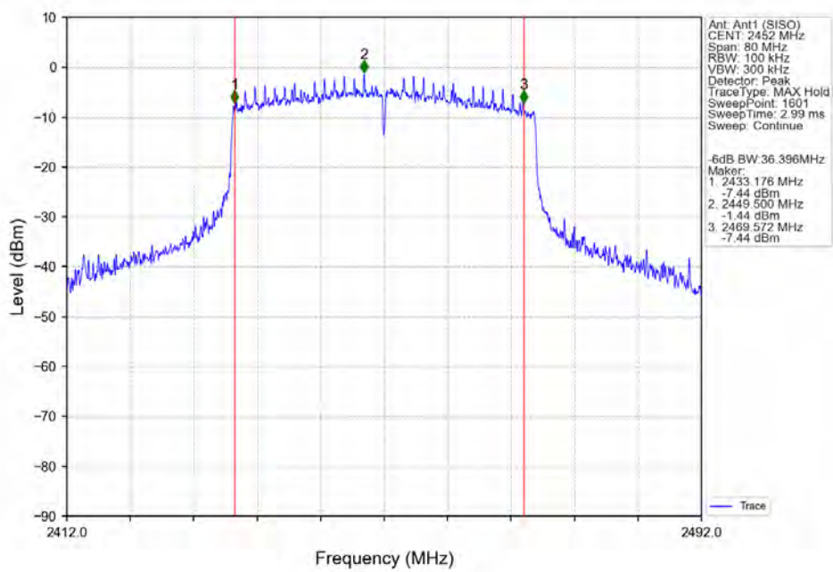
802.11ax(HE40)_HCH_2452MHz_RU484_Left_Ant1 (SISO)_NTNV
