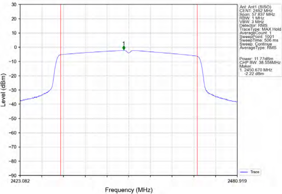
802.11ax(HE40)_HCH_2452MHz_RU484_Left_Ant1 (SISO)_NTNV
