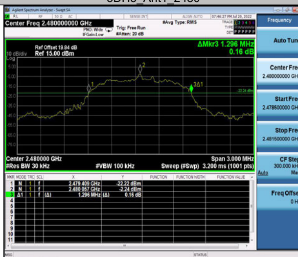
3DH5 Ant1 2480
