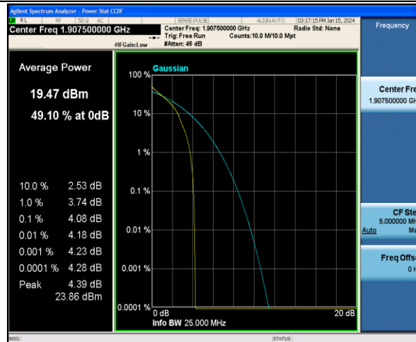
Band2-5MHz-QPSK-19175-1RB#0-PASS
