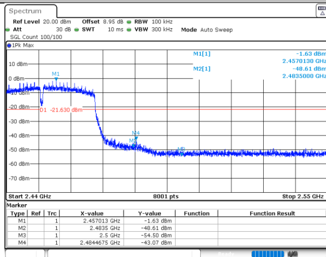
11N40MIMO_Ant2_High_2452
