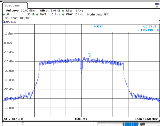
11N40MIMO_Ant2_2437
