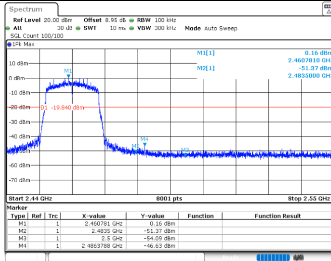
11N20MIMO_Ant2_High_2462
