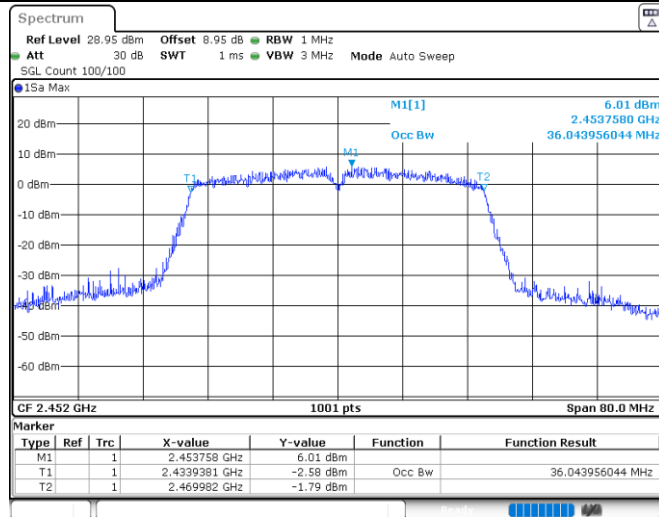
11N40MIMO_Ant2_2452
