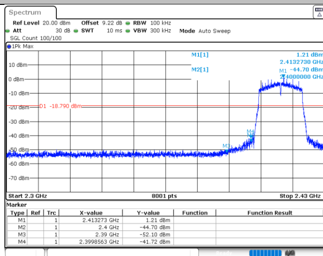
11N20MIMO_Ant1_Low_2412
