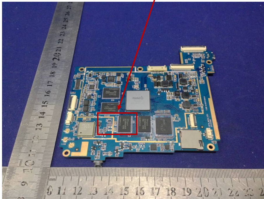
WIFI&BT&GPS Module
